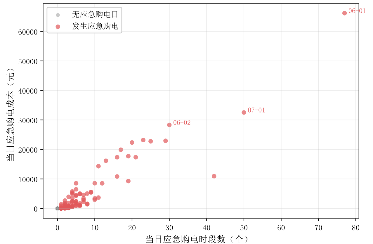
(d) 应急时段数与当日应急购电成本
