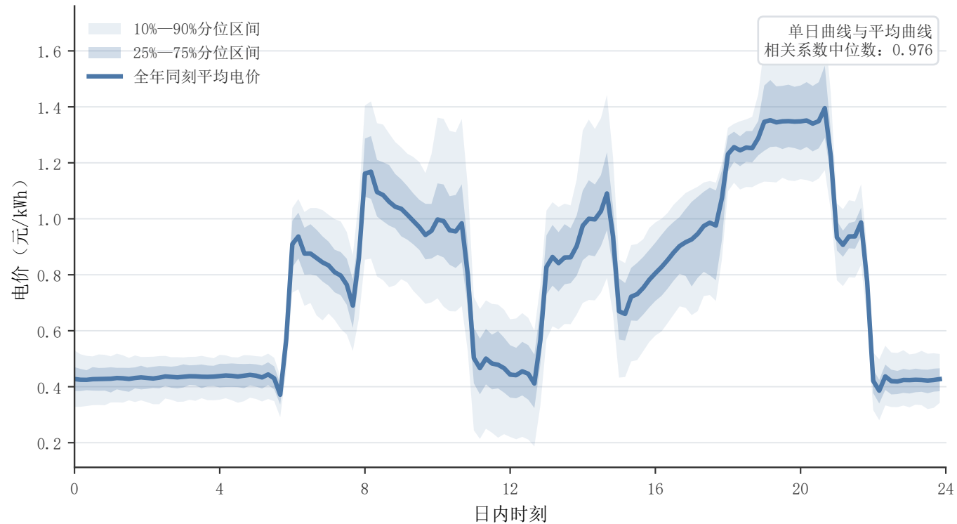
附件4电价的日内形态与跨日波动区间
