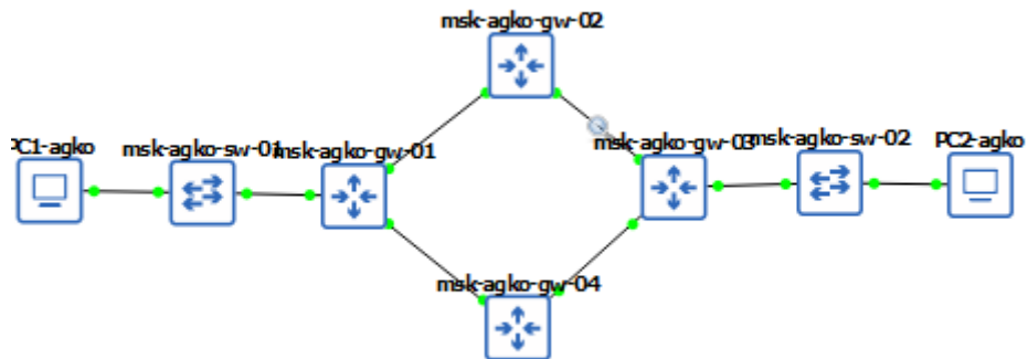
Рисунок 2: Топология сети в GNS3
