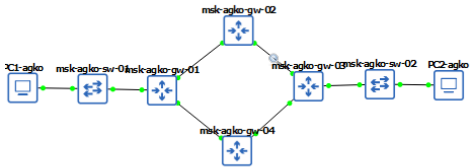
2.2: GNS3
