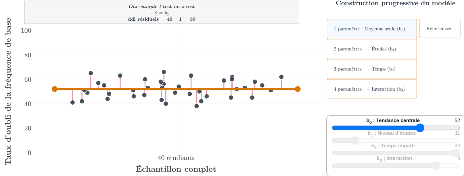
Figure 10: Construction progressive d'un modèle, du one-sample t -test à l'ANOVA factorielle 2 \times 2 .
