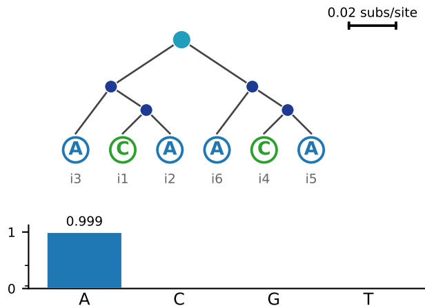
(d) Homoplastic (C on two clades)
