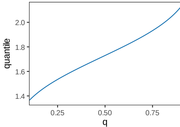
Quantile function
