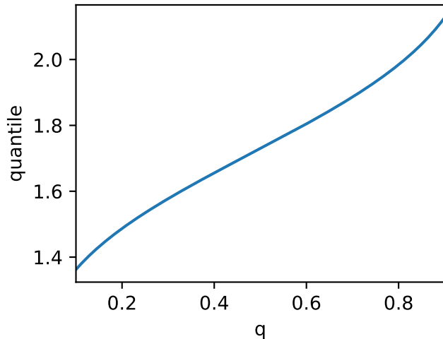
Quantile function
