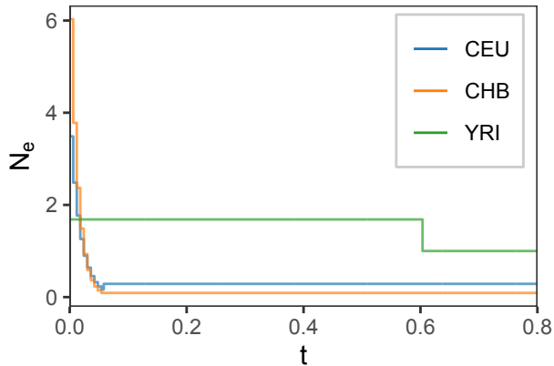
Population size trajectory
