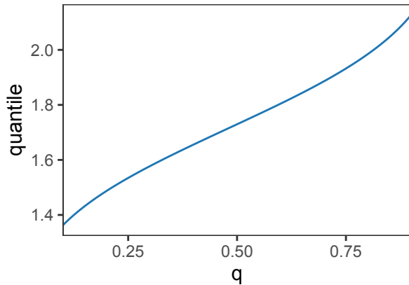
Quantile function
