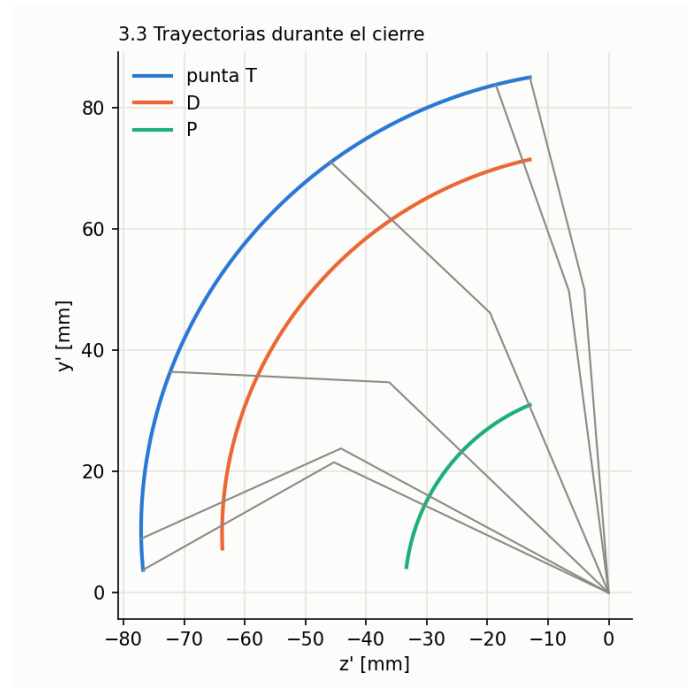
Figura 17: Trayectorias de P, D y T y posturas intermedias del dedo.
