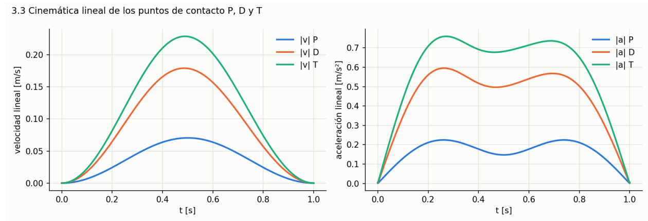
Figura 16: Velocidad y aceleración lineal de los puntos de contacto.
