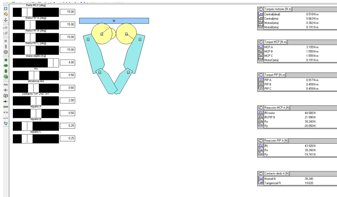
Figura 23: Prueba Power plano V2.4 en Working Model 2D (contacto en D, reparto 50/25/25).
