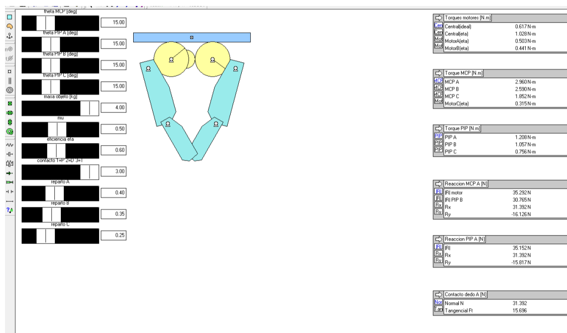
Figura 24: Prueba Carga desigual en Working Model 2D (contacto en T, reparto 40/35/25).
