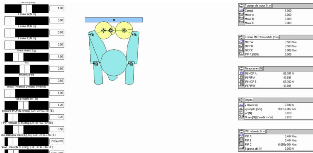
Figura 25: Modelo dinámico sosteniendo un objeto de 1 kg.
