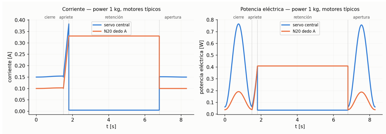
Figura 19: Corriente y potencia eléctrica del servo central y del N20 del dedo A durante un ciclo (power 1 kg).
