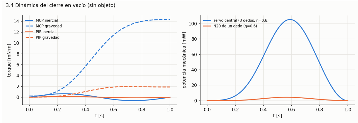
Figura 18: Torques inerciales y gravitacionales y potencia de los motores durante el cierre.
