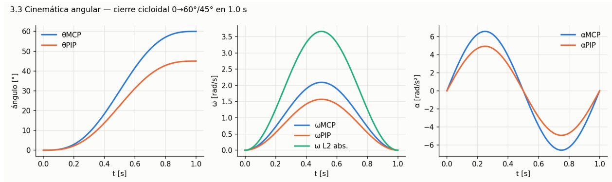
Figura 15: Posición, velocidad y aceleración angular durante el cierre.
