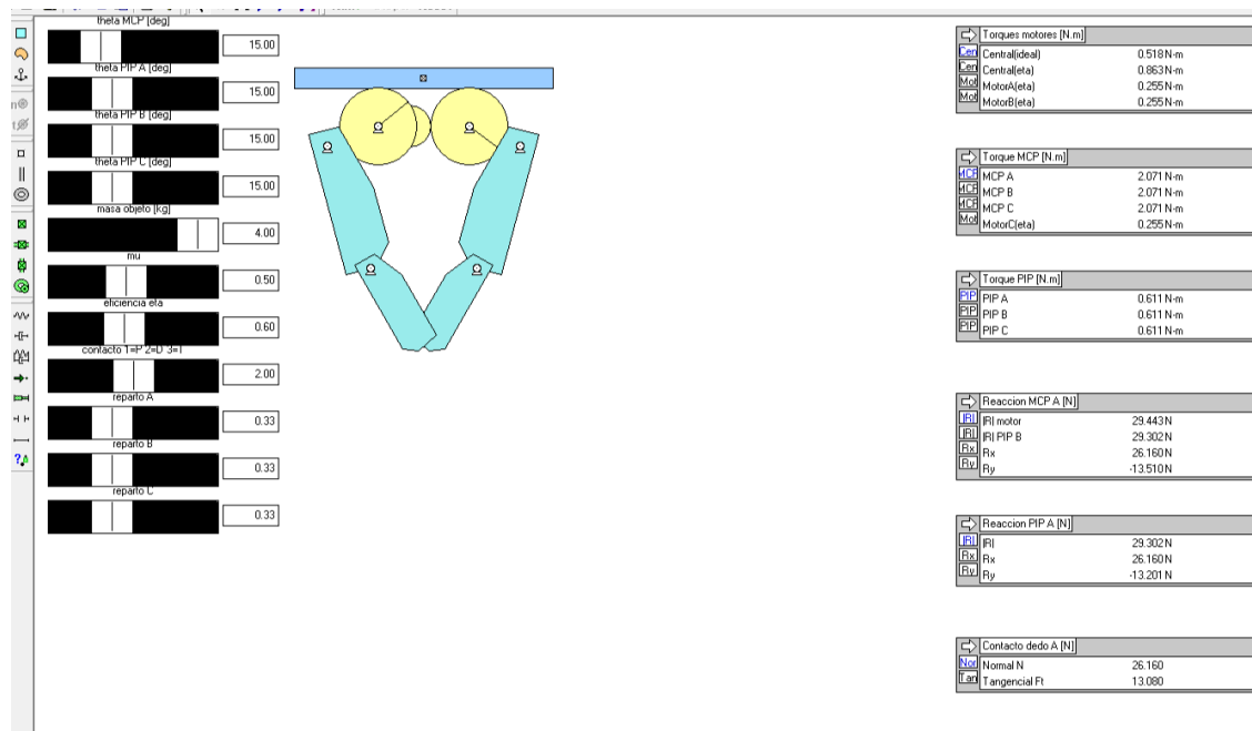
Figura 22: Prueba Power 120° en Working Model 2D (contacto en D, reparto igual).
