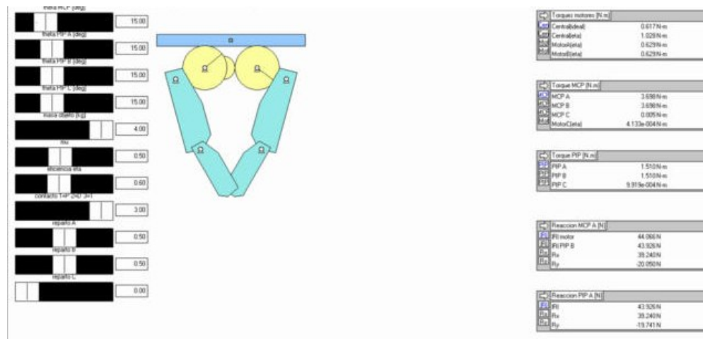
Figura 20: Modelo estático en Working Model 2D.
