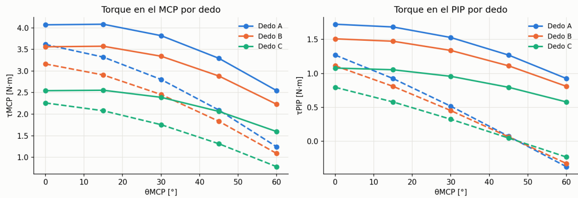
Figura 16. Torques en el MCP y el PIP de cada dedo contra \theta_{MCP} (carga desigual, contacto en T, 3.5 kg, \mu = 0.3 ).
