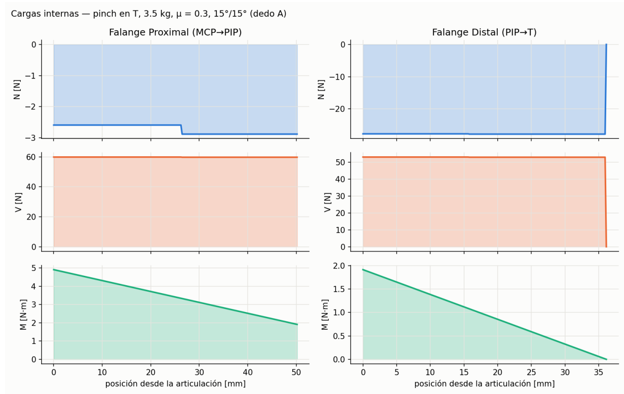
Figura 17: Fuerza normal, cortante y momento flector a lo largo de cada falange (pinch en la punta, dedo A).
