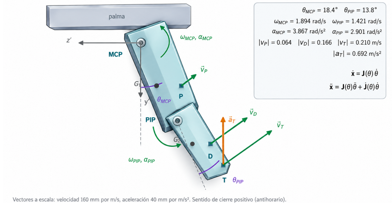
Figura 20: Diagrama cinemático del dedo en t = 0.4 s del cierre cicloidal. Diagrama generado con el modelo y mejorado gráficamente con IA; los valores se verificaron contra el cálculo.
