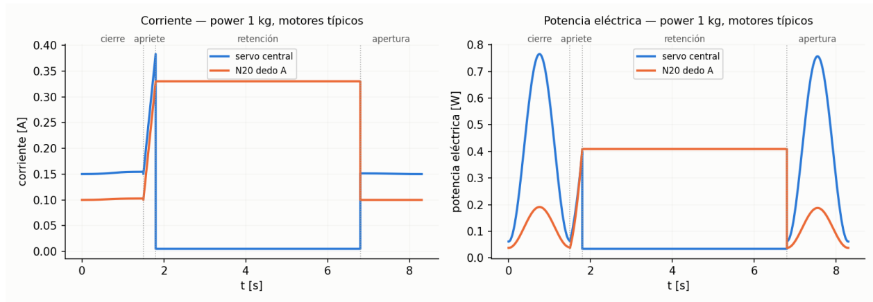
Figura 26: Corriente y potencia eléctrica del servo central y del N20 del dedo A durante un ciclo (power 1 kg).
