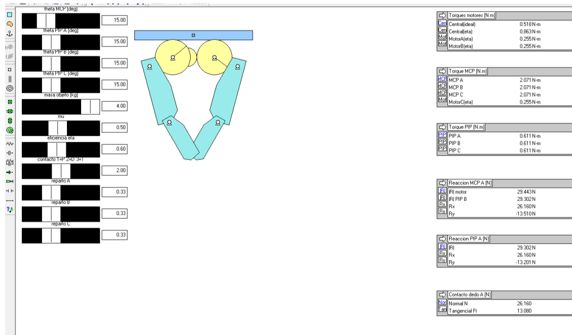
Figura 29: Prueba Power 120° en Working Model 2D (contacto en D, reparto igual).
