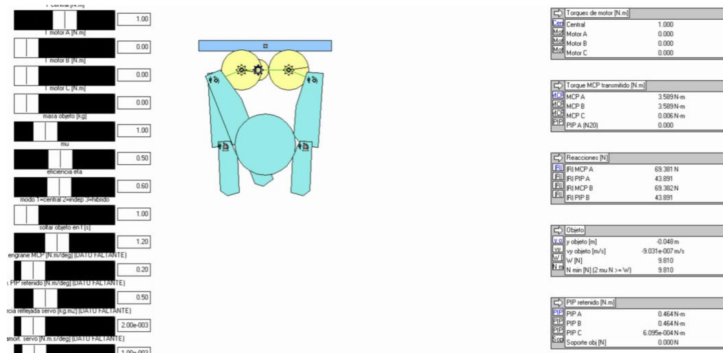
Figura 32: Modelo dinámico sosteniendo un objeto de 1 kg.
