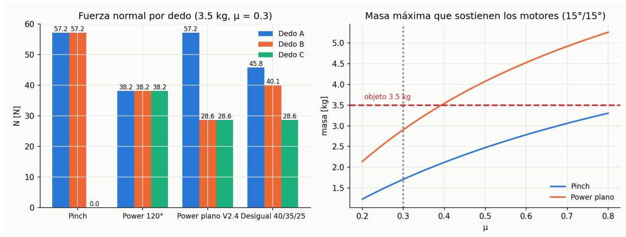
Figura 18: Fuerza normal por dedo y masa máxima que sostienen los motores en función de \mu .
