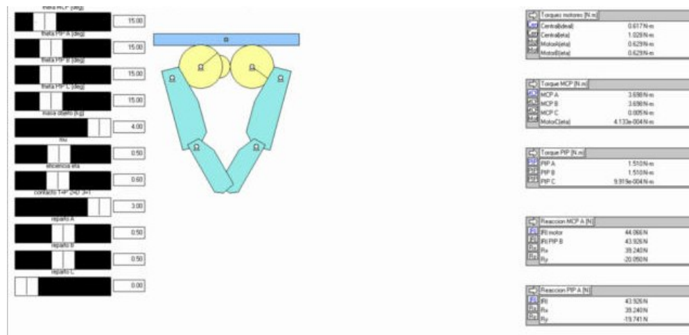
Figura 9: Modelo estático en Working Model 2D.
