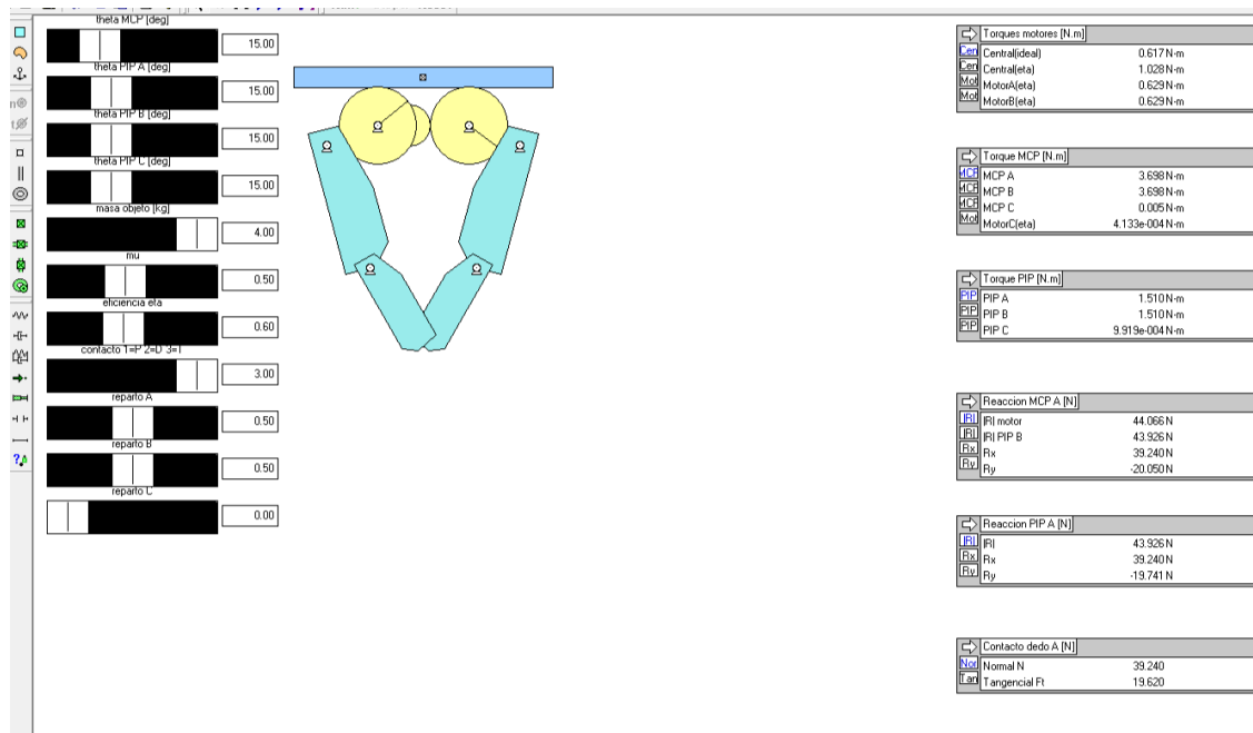
Figura 10: Prueba Pinch en Working Model 2D (contacto en T, reparto 50/50/0).
