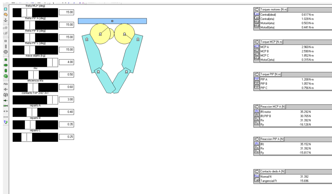
Figura 13: Prueba Carga desigual en Working Model 2D (contacto en T, reparto 40/35/25).
