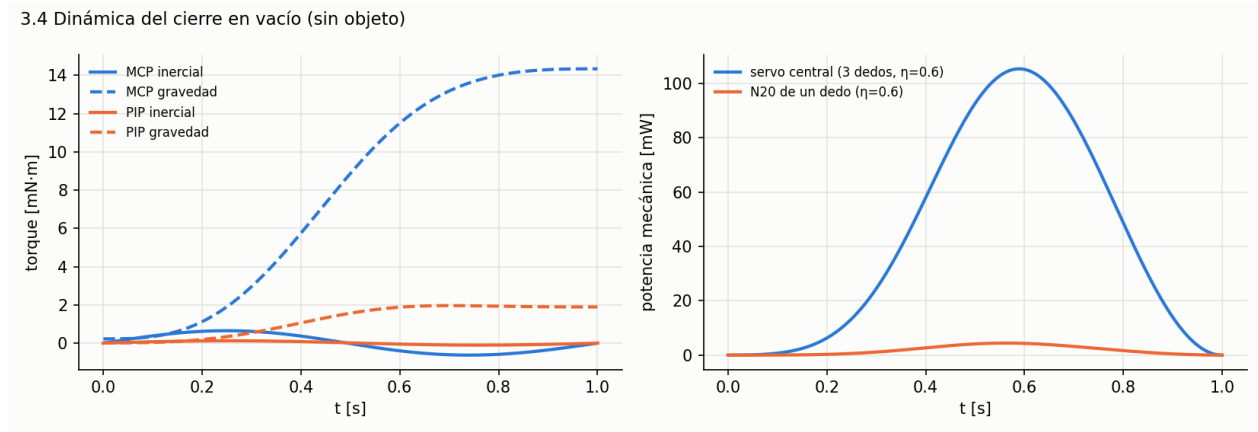
Figura 8: Torques inerciales y gravitacionales y potencia de los motores durante el cierre.
