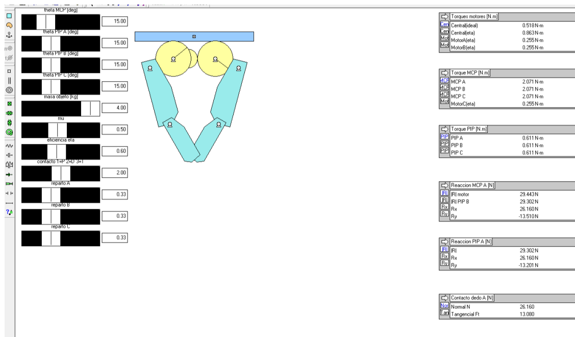
Figura 11: Prueba Power 120° en Working Model 2D (contacto en D, reparto igual).
