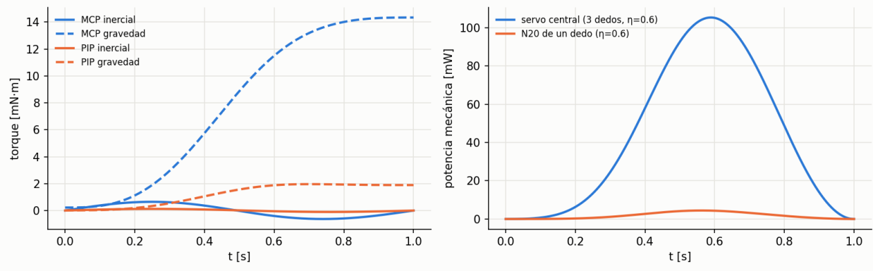
Figura 28: Torques inerciales y gravitacionales y potencia de los motores durante el cierre.
