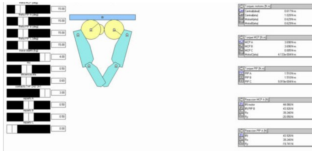
Figura 30: Modelo estático en Working Model 2D.
