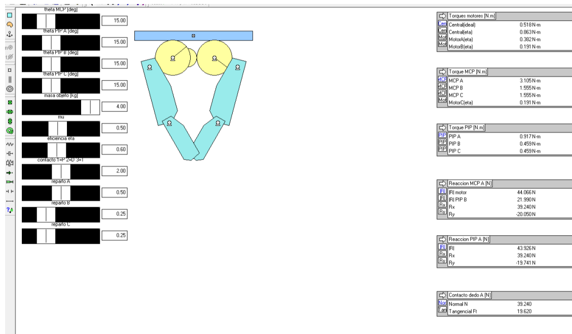
Figura 33: Prueba Power plano V2.4 en Working Model 2D (contacto en D, reparto 50/25/25).
