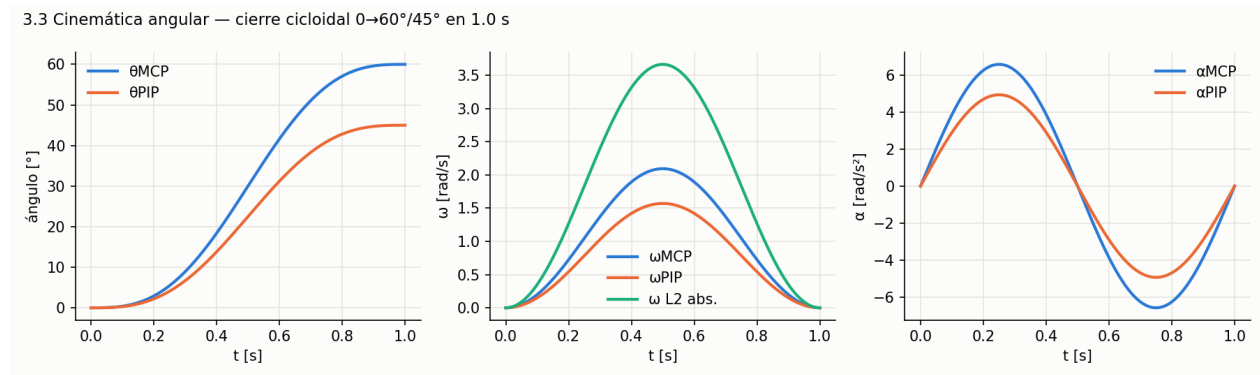
Figura 24: Posición, velocidad y aceleración angular durante el cierre.
