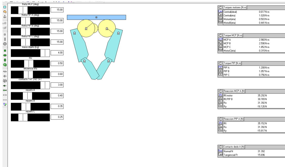
Figura 34: Prueba Carga desigual en Working Model 2D (contacto en T, reparto 40/35/25).
