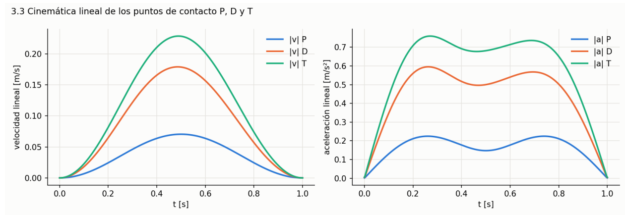
Figura 25: Velocidad y aceleración lineal de los puntos de contacto.
