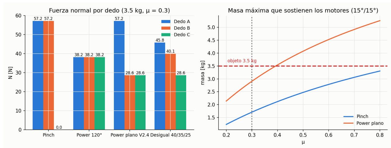
Figura 21: Fuerza normal por dedo y masa máxima que sostienen los motores en función de \mu .
