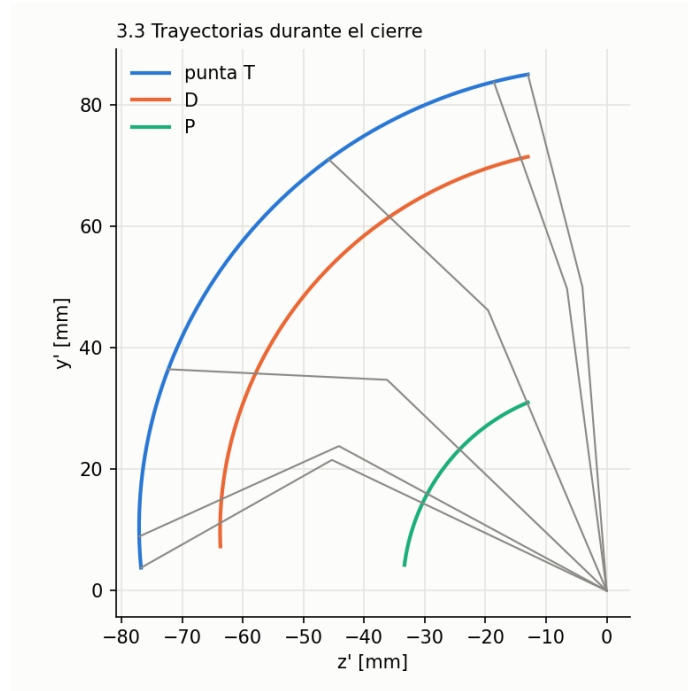
Figura 26: Trayectorias de P, D y T y posturas intermedias del dedo.
