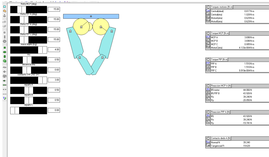
Figura 31: Prueba Pinch en Working Model 2D (contacto en T, reparto 50/50/0).
