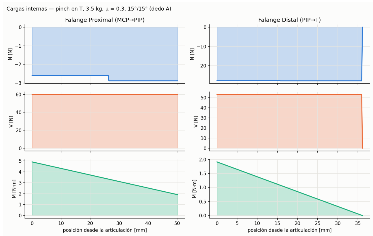
Figura 21: Fuerza normal, cortante y momento flector a lo largo de cada falange (pinch en la punta, dedo A).
