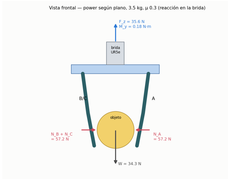
Figura 19: Diagrama de cuerpo libre en vista frontal con 3.5 kg y \mu = 0.3 .
