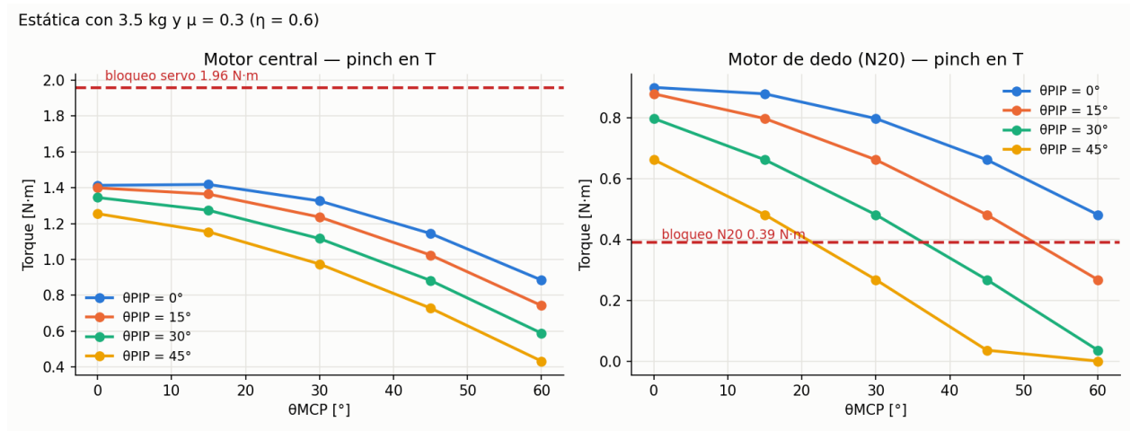
Figura 15: Torques del motor central y del N20 en pinch en la punta, con los pares de bloqueo típicos.
