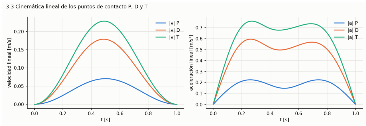
Figura 26: Velocidad y aceleración lineal de los puntos de contacto.
