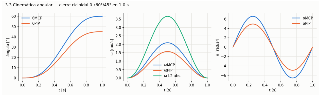
Figura 25: Posición, velocidad y aceleración angular durante el cierre.
