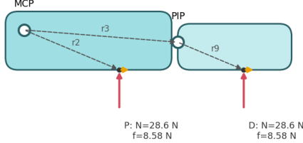
Figura 20: Diagrama de cuerpo libre del dedo recto en los cuatro casos de agarre (3.5 kg, \mu = 0.3 ).
