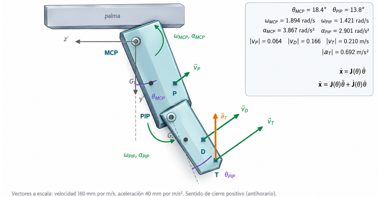
Figura 24: Diagrama cinemático del dedo en t = 0.4 s del cierre cicloidal. Diagrama generado con el modelo y mejorado gráficamente con IA; los valores se verificaron contra el cálculo.
