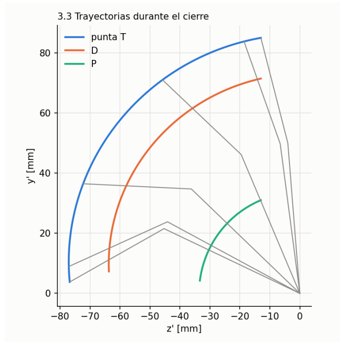
Figura 27: Trayectorias de P, D y T y posturas intermedias del dedo.
