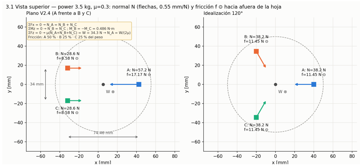
Figura 18: Vista superior con 3.5 kg y \mu = 0.3 : normales en el plano y fricción hacia afuera de la hoja.
