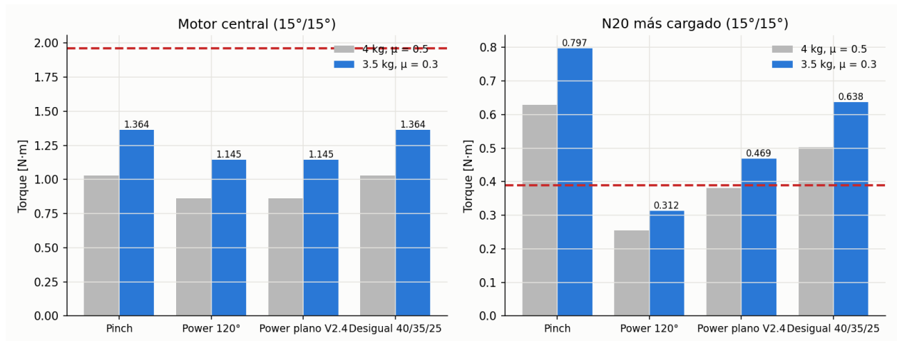
Figura 16: Torques de motor de los dos casos de diseño en la postura 15°/15°.
