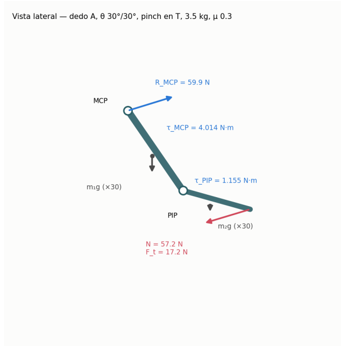
Figura 17: Diagrama de cuerpo libre en vista lateral del dedo A, 3.5 kg y \mu = 0.3 .
