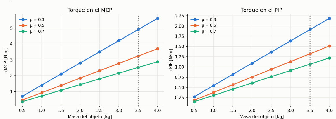
Figura 22. Torques en el MCP y el PIP del dedo A contra la masa del objeto, para \mu = 0.3, 0.5 y 0.7 (pinch en T, 15^\circ/15^\circ ).
