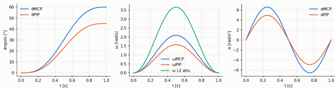
Figura 25. Posición, velocidad y aceleración angular durante el cierre.
