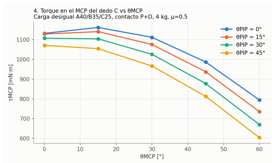
Figura 8. Torque en el MCP del dedo C contra \theta_{MCP} .
