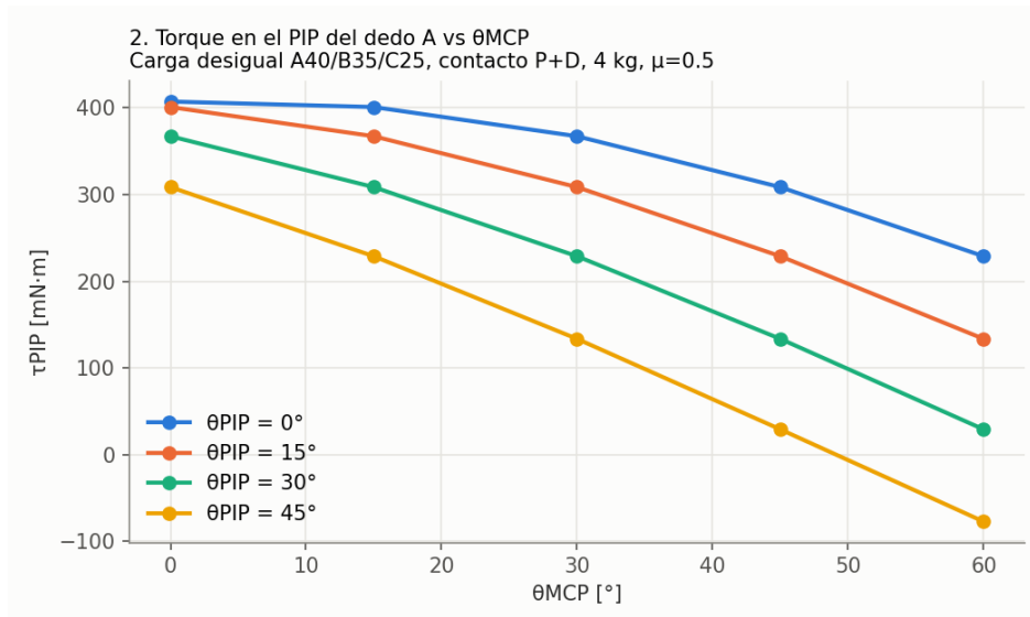
Figura 6. Torque en el PIP del dedo A contra \theta_{MCP} .
