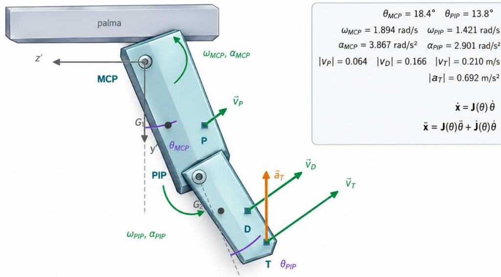
Figura 24. Diagrama cinemático del dedo en t = 0.4 s del cierre cicloidal. Diagrama generado con el modelo y mejorado gráficamente con IA; los valores se verificaron contra el cálculo.
