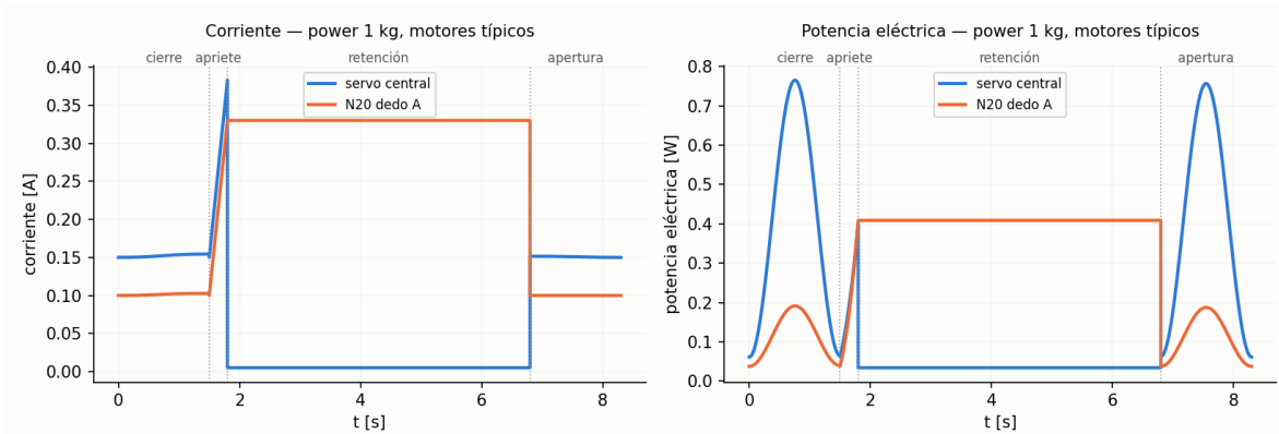
Figura 30. Corriente y potencia eléctrica del servo central y del N20 del dedo A durante un ciclo (power 1 kg).
