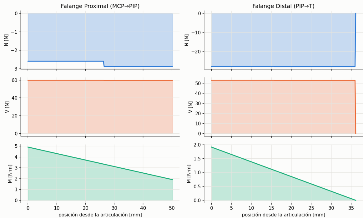
Figura 21. Fuerza normal, cortante y momento flector a lo largo de cada falange (pinch en la punta, dedo A).
