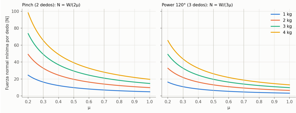
Figura 11. Fuerza normal mínima por dedo contra el coeficiente de fricción.
