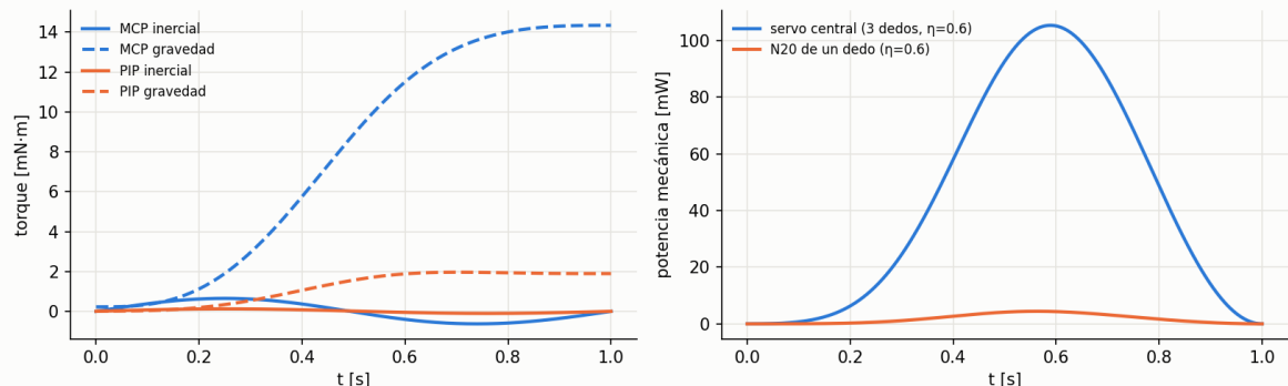
Figura 29. Torques inerciales y gravitacionales y potencia de los motores durante el cierre.
