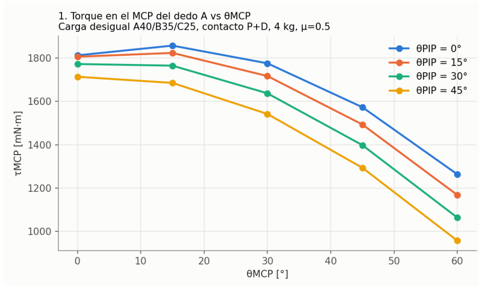
Figura 5. Torque en el MCP del dedo A contra \theta_{MCP} (carga desigual, contacto P+D, 4 kg, \mu = 0.5 ).
