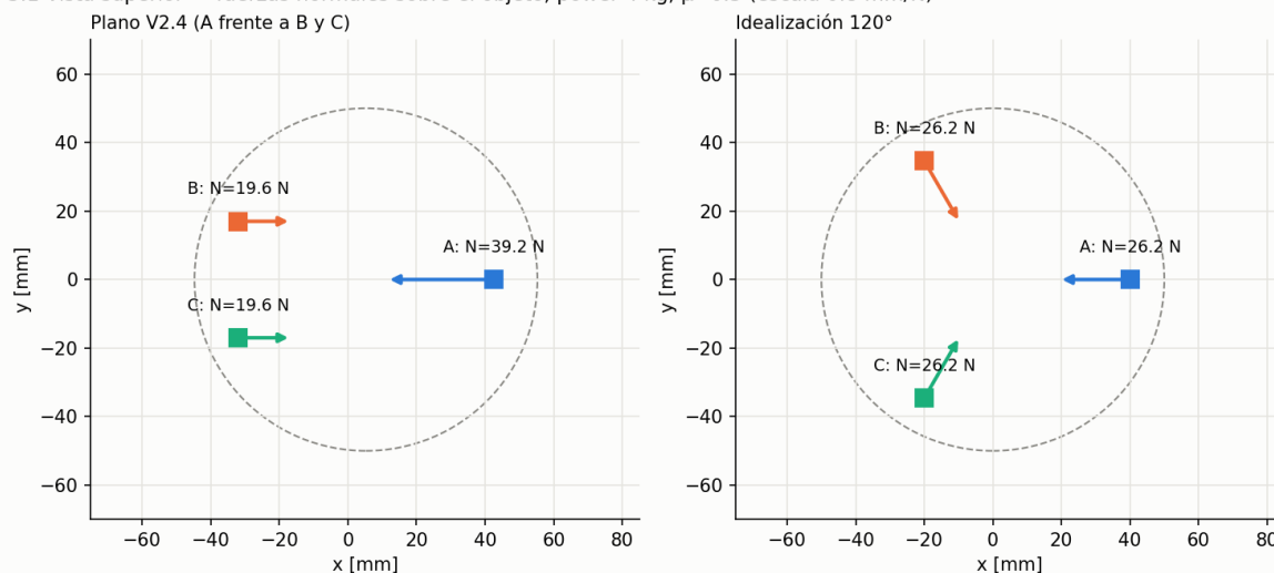
Figura 3. Fuerzas normales en vista superior según el plano y con la idealización a 120°.
