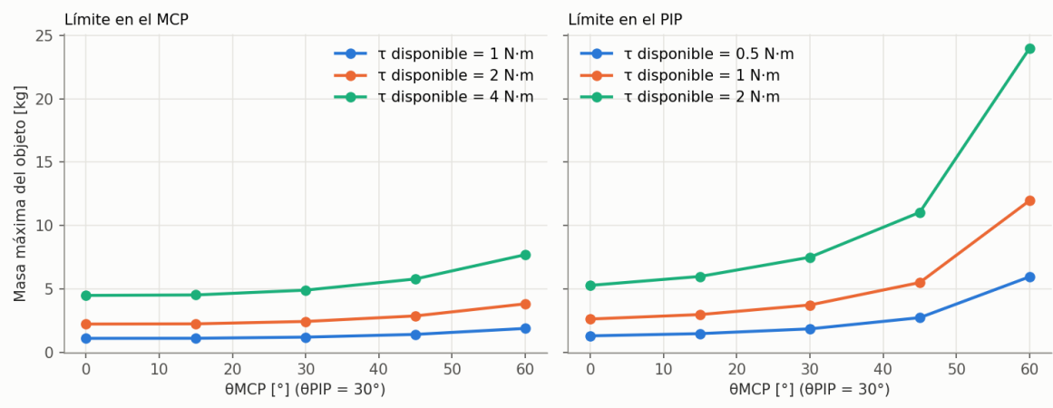
Figura 12. Masa máxima sostenible según el torque disponible en cada articulación.
