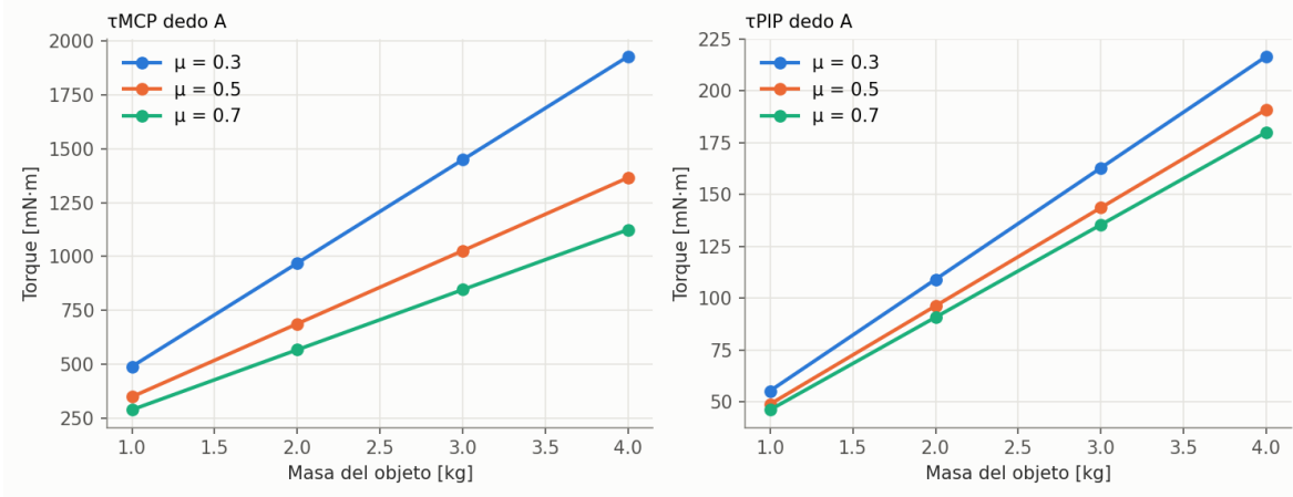
Figura 13. Torques en las articulaciones del dedo A contra la masa del objeto.
