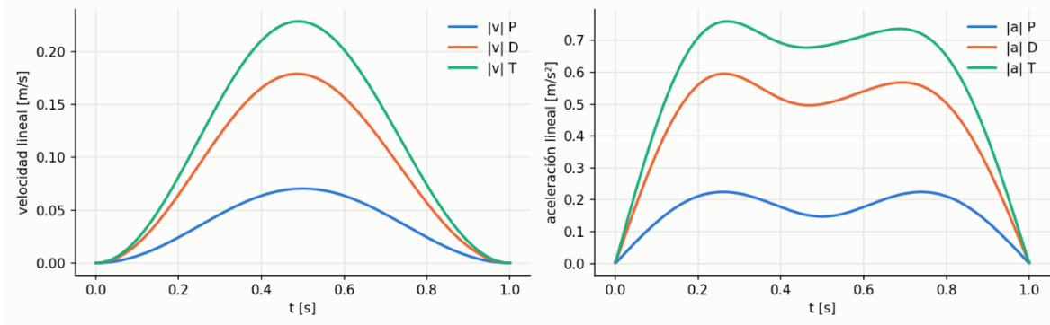
Figura 26. Velocidad y aceleración lineal de los puntos de contacto.
