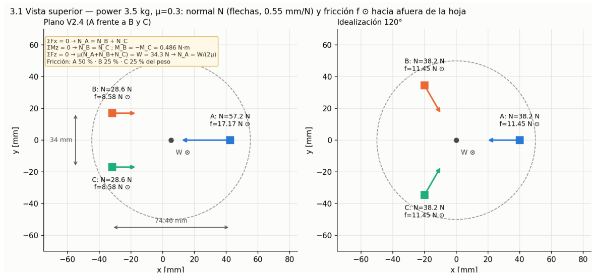
Figura 18. Vista superior con 3.5 kg y \mu = 0.3 : normales en el plano y fricción hacia afuera de la hoja.
