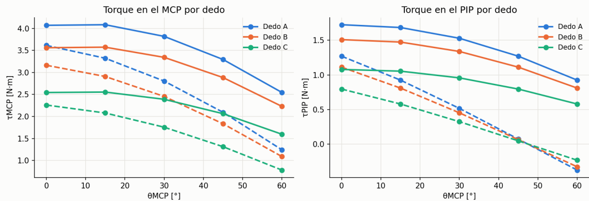
Figura 16. Torques en el MCP y el PIP de cada dedo contra \theta_{MCP} (carga desigual, contacto en T, 3.5 kg, \mu = 0.3 ).
