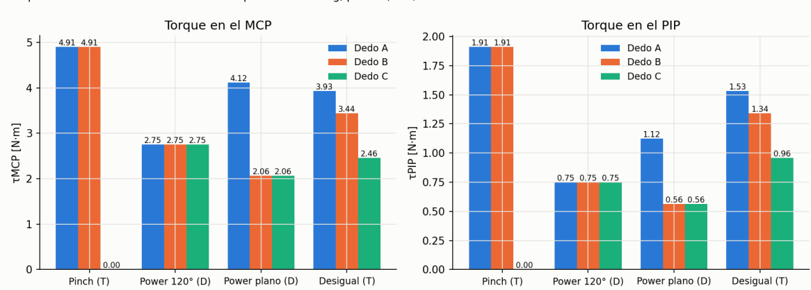
Figura 15. Torques en las articulaciones de cada dedo en las cuatro pruebas (3.5 kg, \mu = 0.3 , 15°/15°).
