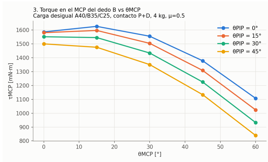
Figura 7. Torque en el MCP del dedo B contra \theta_{MCP} .
