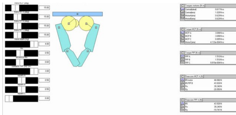
Figura 10: Modelo estático en Working Model 2D.
