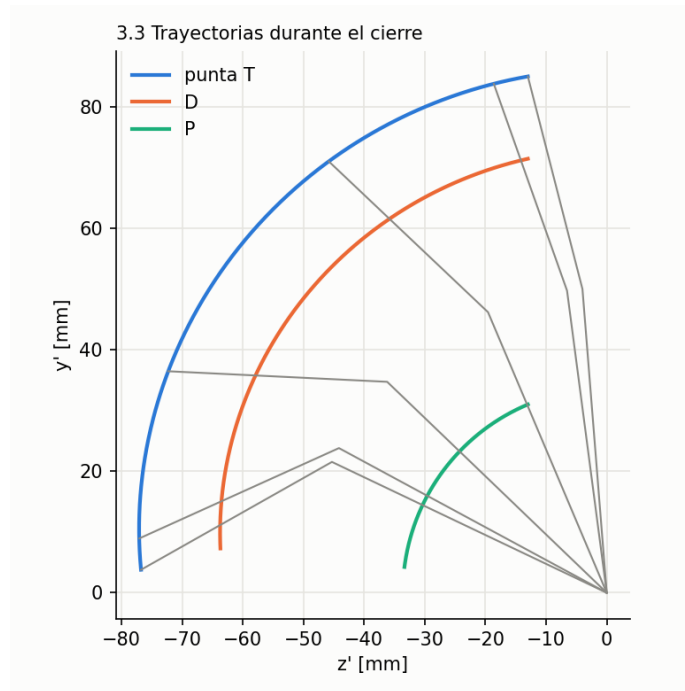
Figura 7: Trayectorias de P, D y T y posturas intermedias del dedo.
