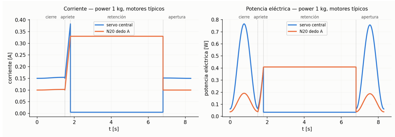
Figura 9: Corriente y potencia eléctrica del servo central y del N20 del dedo A durante un ciclo (power 1 kg).
