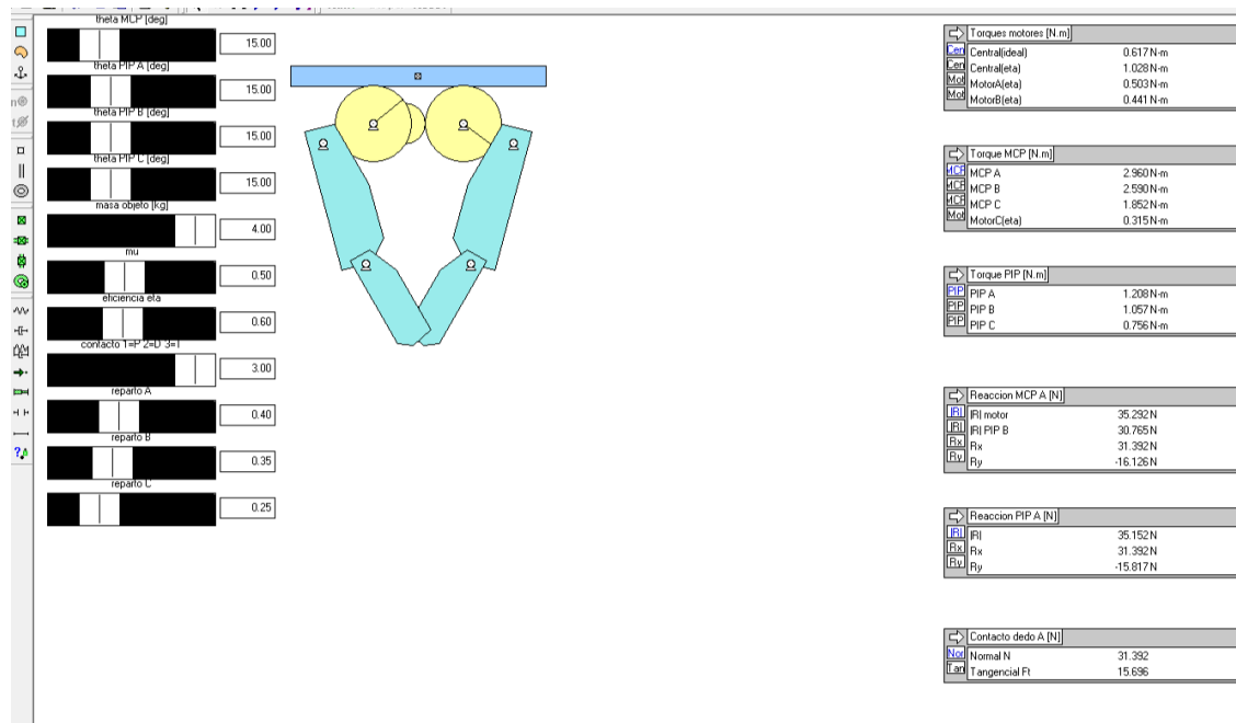
Figura 14: Prueba Carga desigual en Working Model 2D (contacto en T, reparto 40/35/25).
