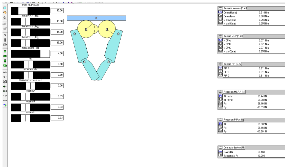
Figura 12: Prueba Power 120° en Working Model 2D (contacto en D, reparto igual).
