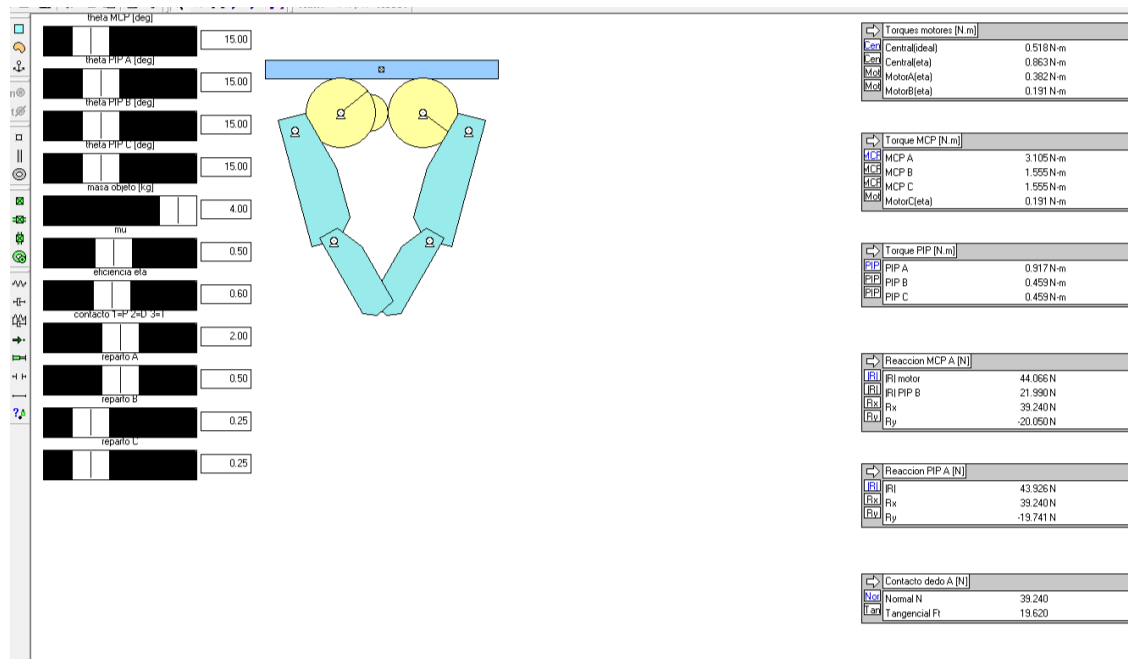
Figura 13: Prueba Power plano V2.4 en Working Model 2D (contacto en D, reparto 50/25/25).
