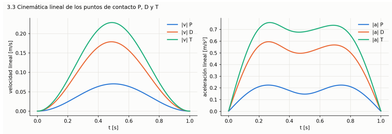
Figura 6: Velocidad y aceleración lineal de los puntos de contacto.
