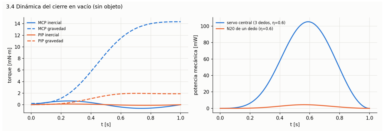
Figura 8: Torques inerciales y gravitacionales y potencia de los motores durante el cierre.
