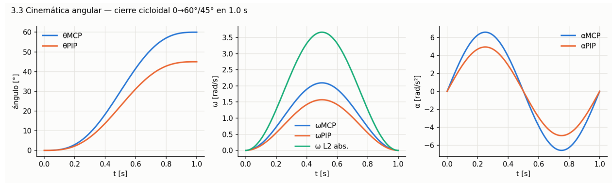
Figura 5: Posición, velocidad y aceleración angular durante el cierre.
