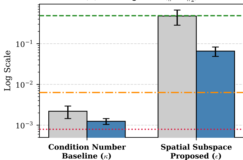
(d) Filter Jitter ( \|\Delta \mathbf{w}\|_2^2 )
