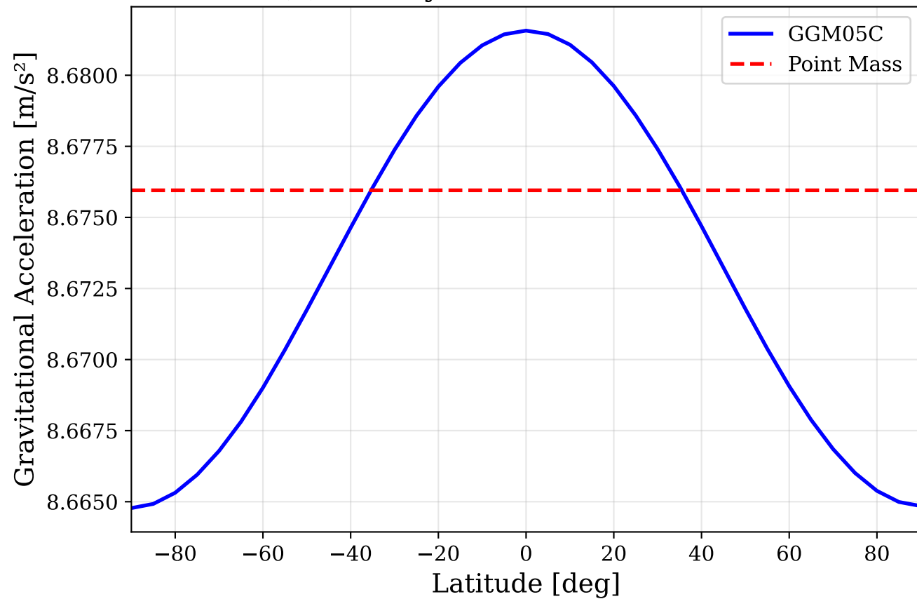
(a) Gravity vs Latitude at 400km
