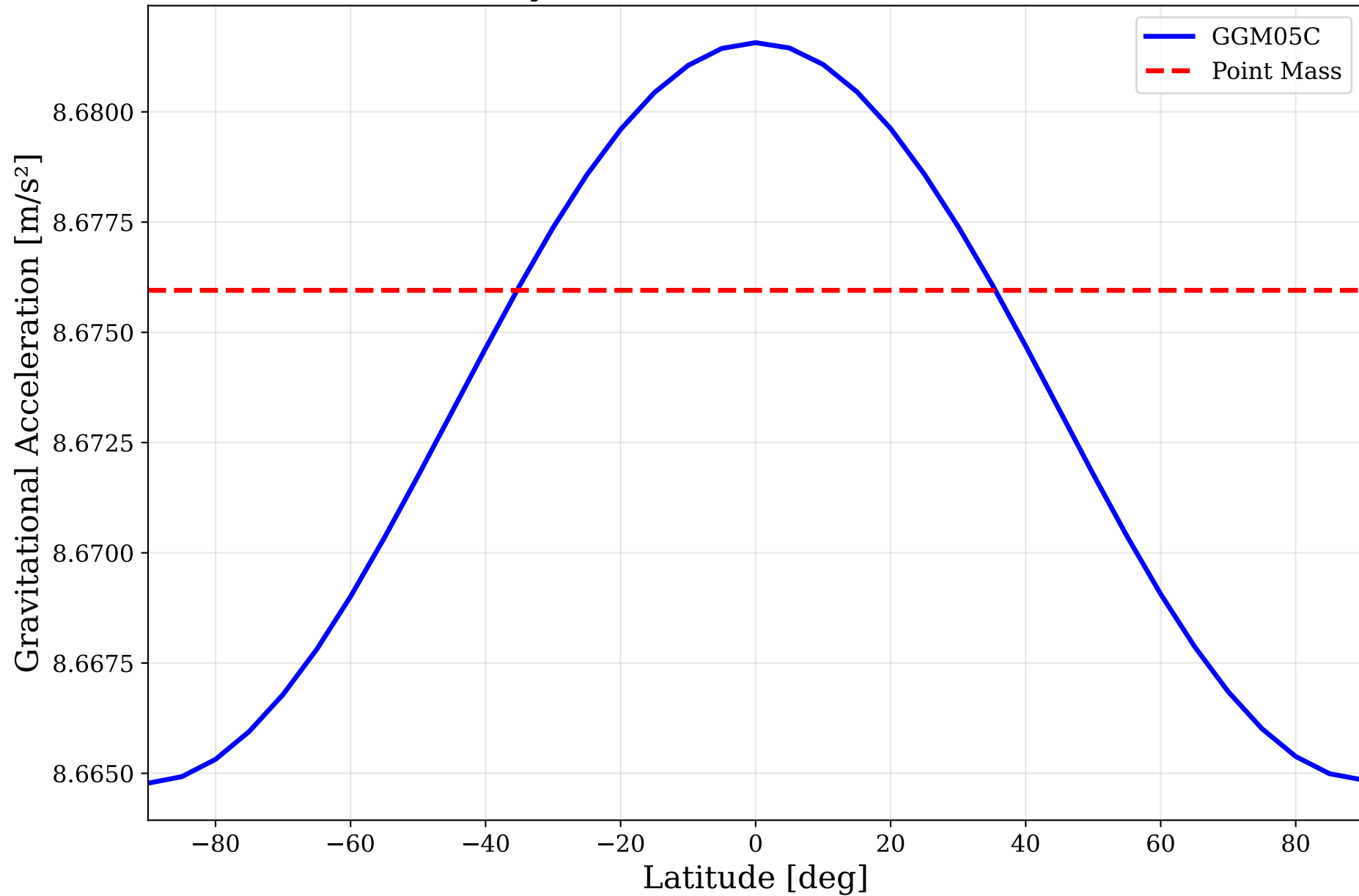
Gravity vs Latitude at 400km Altitude
