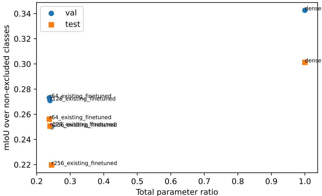
mIoU vs Total parameter ratio
