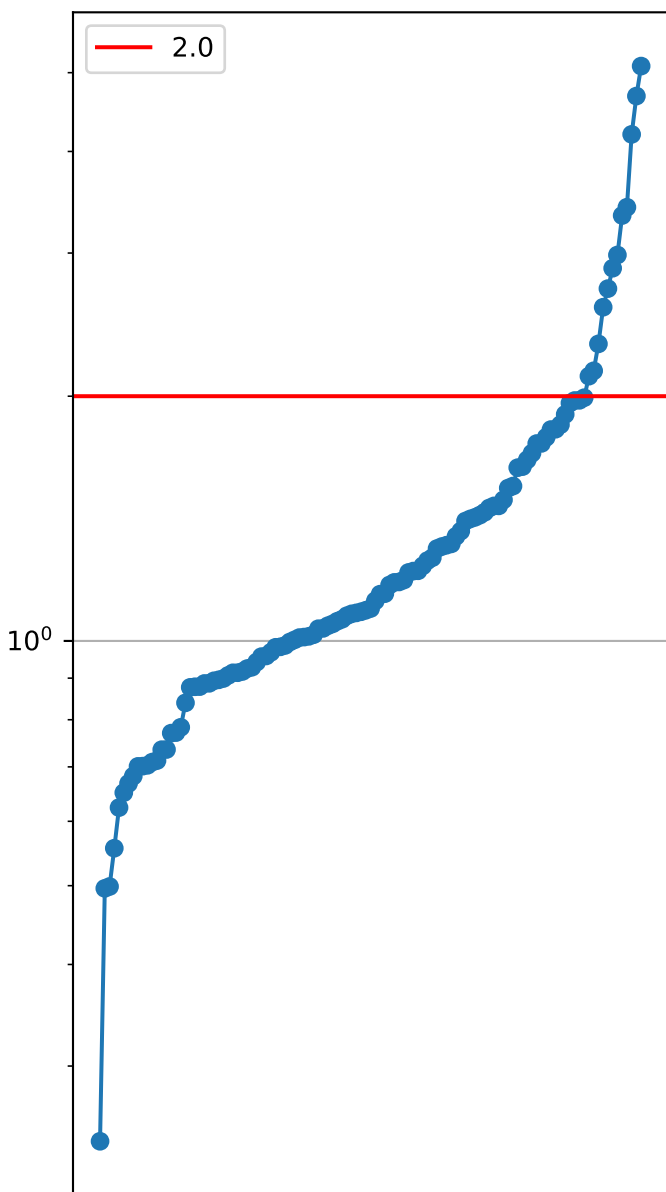
Gecode 2/4 - 115/200 instances
