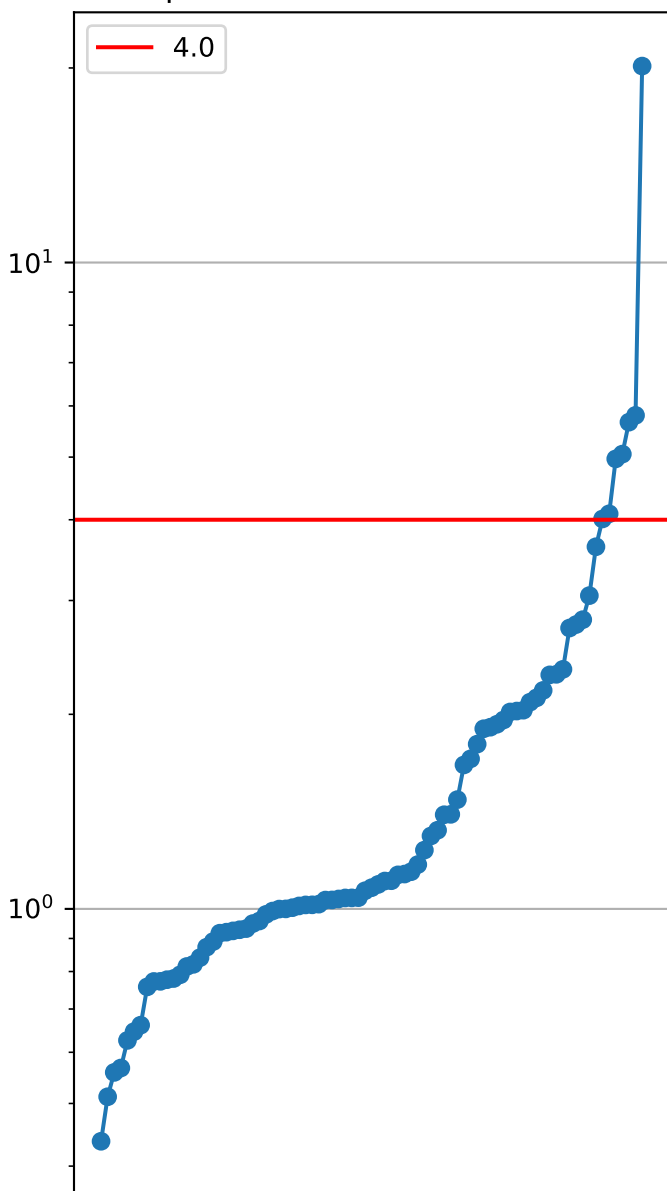
Cplex 2/8 - 83/200 instances
