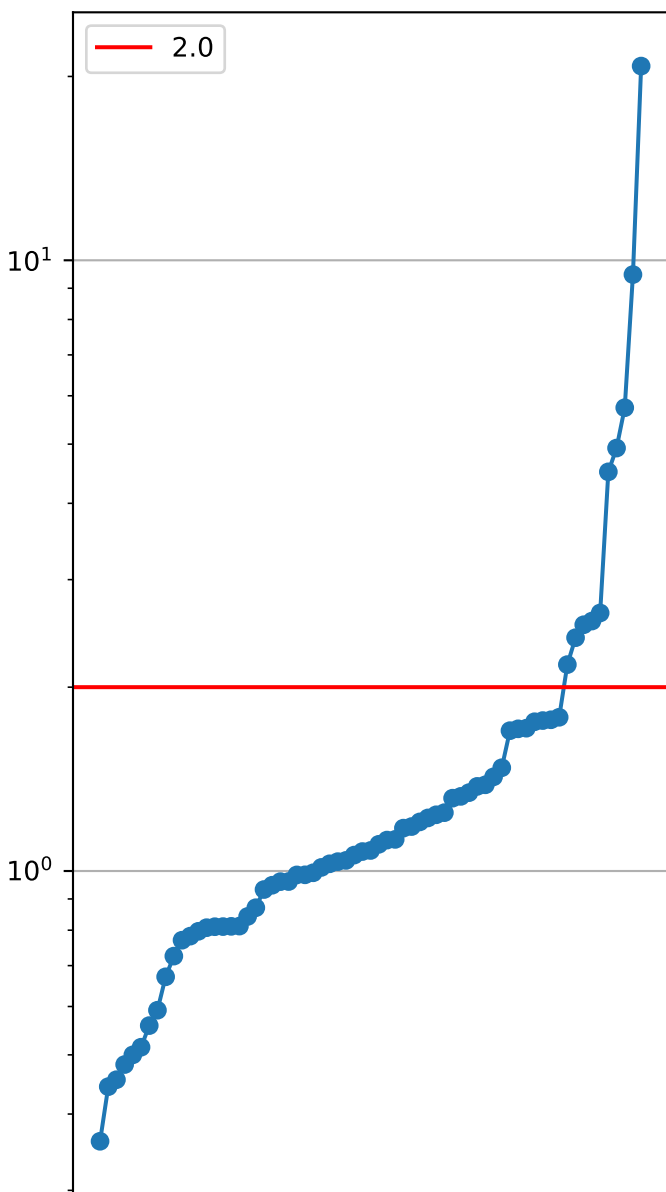
Choco 2/4 - 67/200 instances
