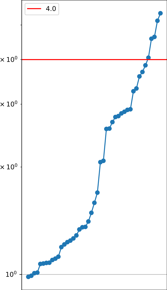
Gecode 1/4 - 45/200 instances
