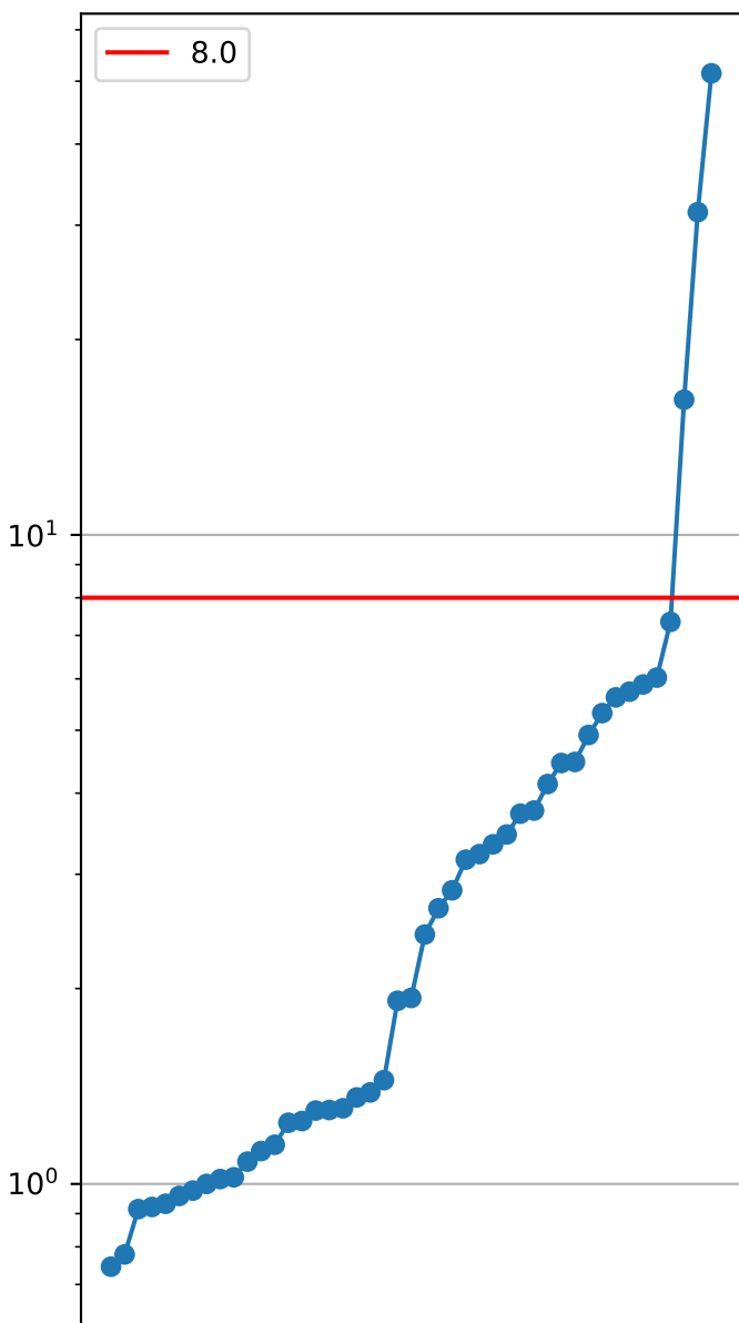
Gecode 1/8 - 45/200 instances
