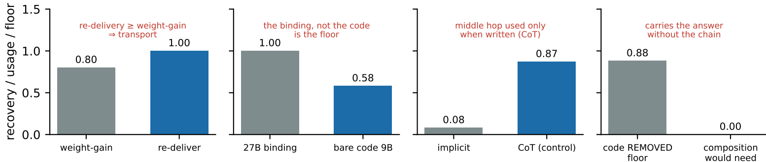
\gamma : attention
