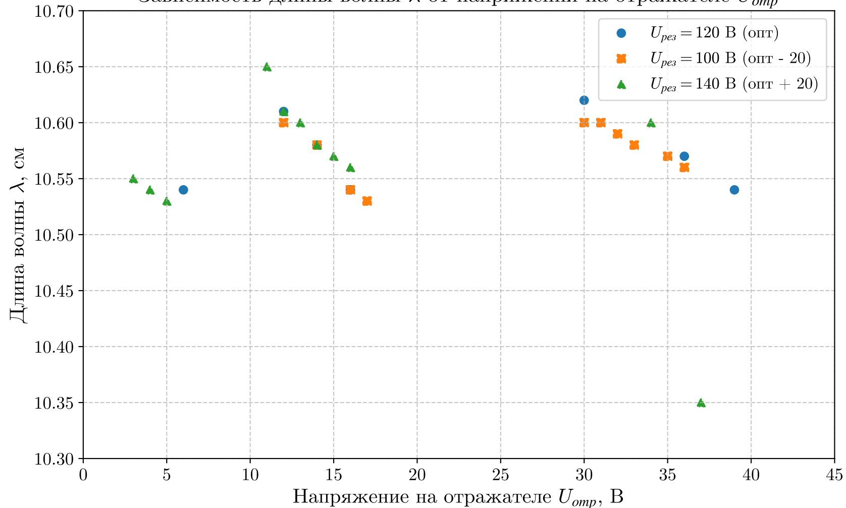
Зависимость длины волны \lambda от напряжения на отражателе U_{отр}
