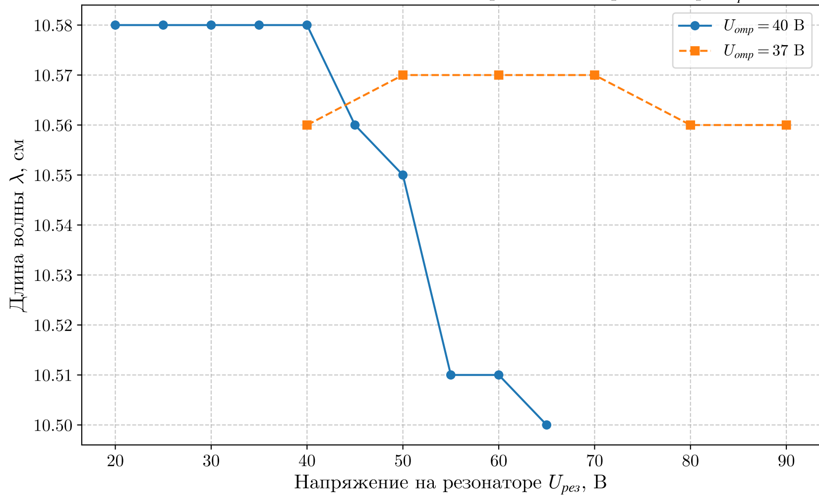
Зависимость длины волны \lambda от напряжения на резонаторе U_{рез}
