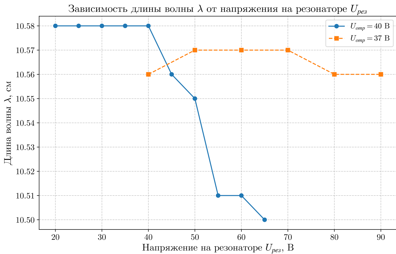
Рис. 7. Зависимость длины волны \lambda от напряжения на резонаторе U_{рез} при различных U_{отр}
