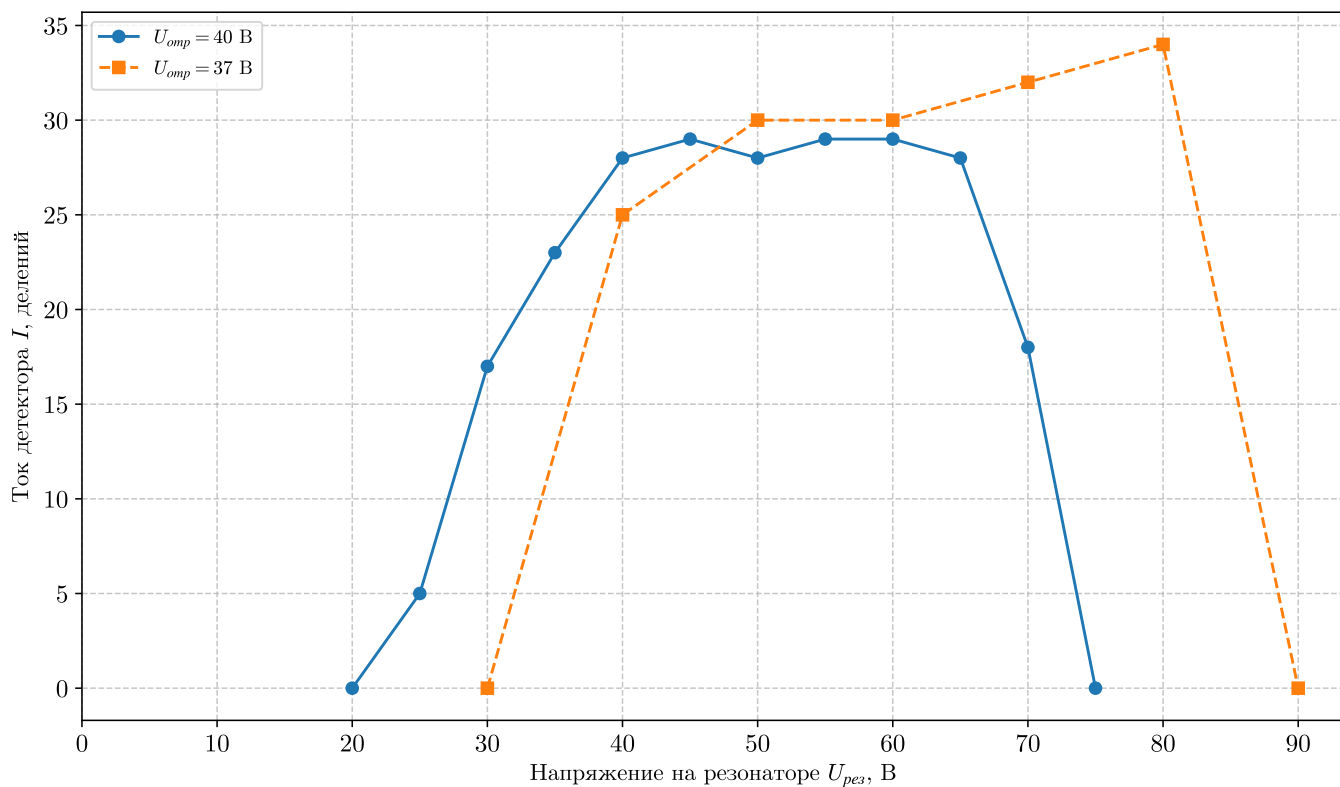
Рис. 6. Зависимости тока детектора I от напряжения на резонаторе U_{рез}
