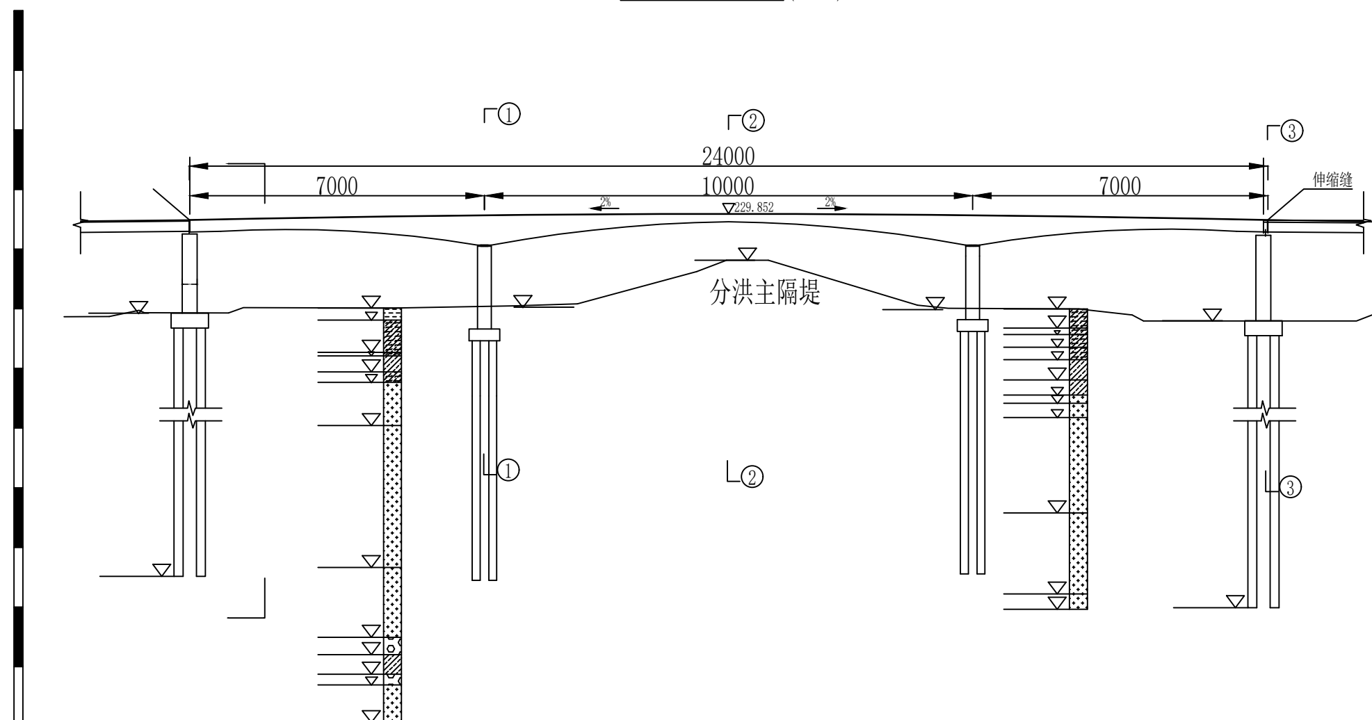
全桥桥型布置图 (1:600)
