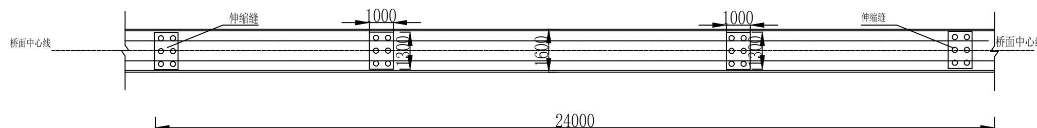
全桥平面布置图 (1:1000)
