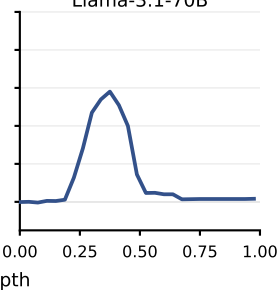
Llama-3.1-70B
