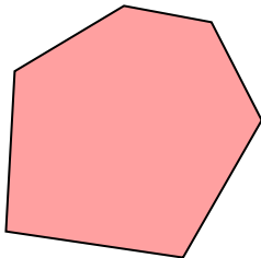
Рис. 3: Выпуклая область
