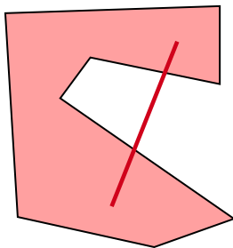
Рис. 4: Невыпуклая область
