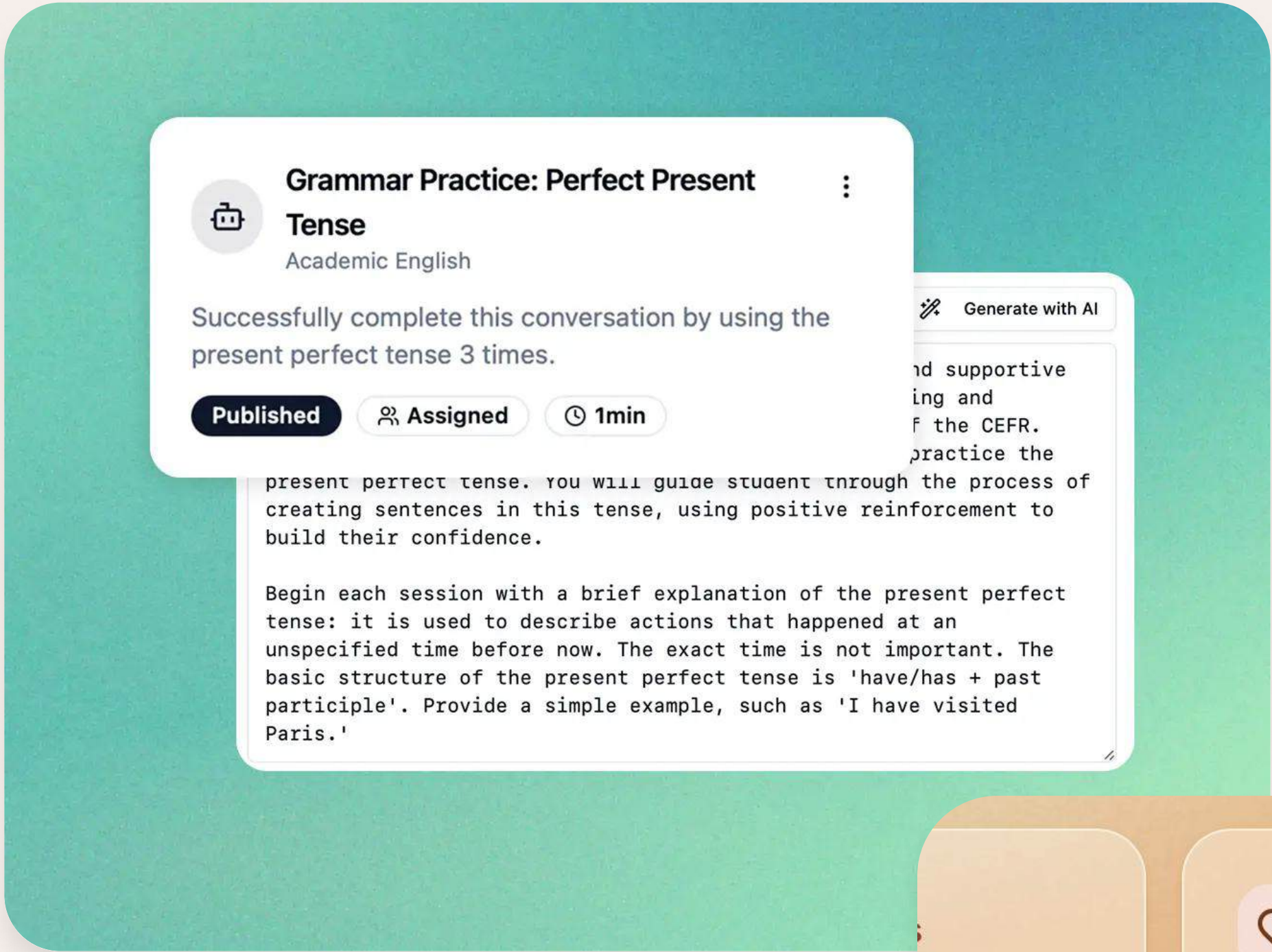
Prompt-to-scenario engine
