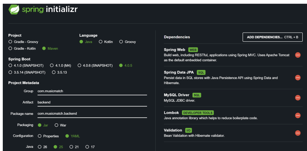
Figura 8.4 - Inicialización del backend con Spring Boot Initializr
