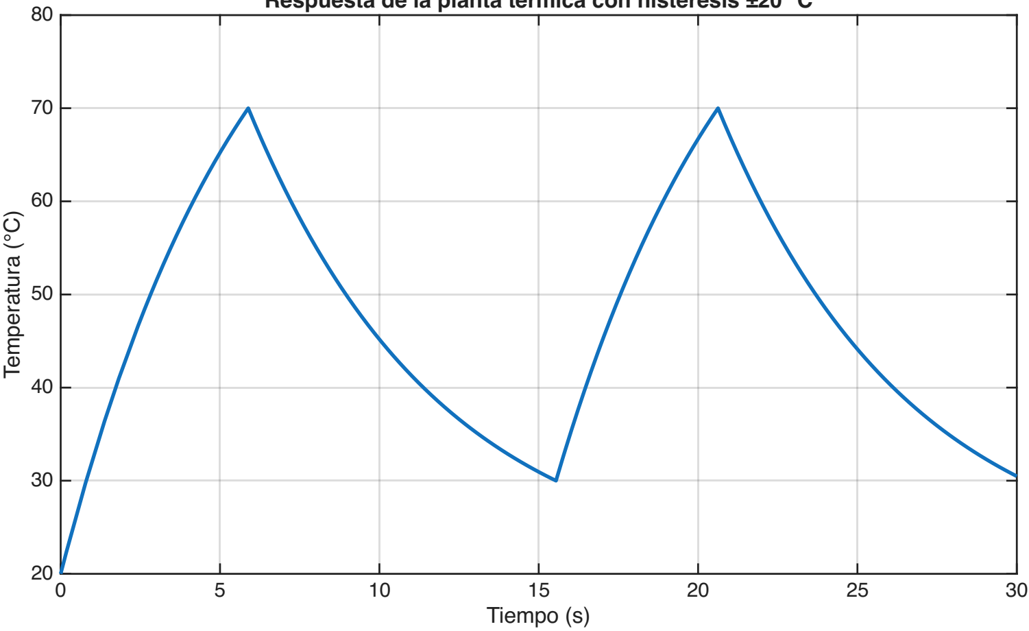
Respuesta de la planta térmica con histéresis \pm 20\text{ }^{\circ}\text{C}
