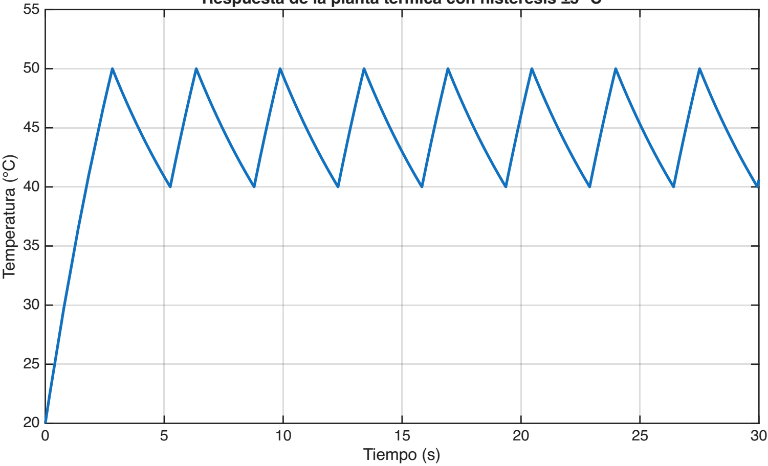
Respuesta de la planta térmica con histéresis \pm 5\text{ }^{\circ}\text{C}
