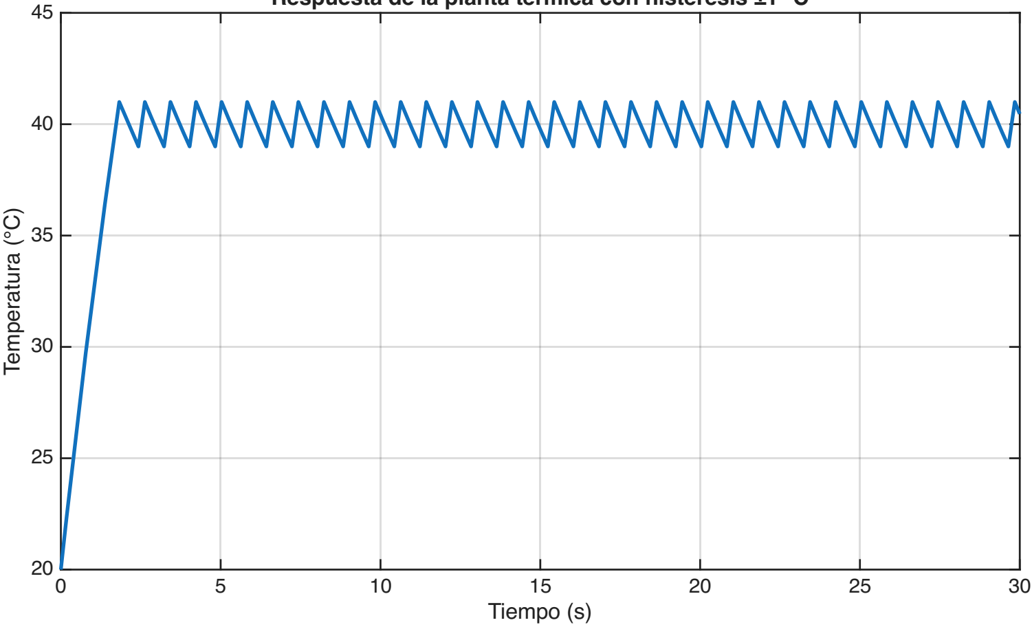
Respuesta de la planta térmica con histéresis \pm 1\text{ }^{\circ}\text{C}
