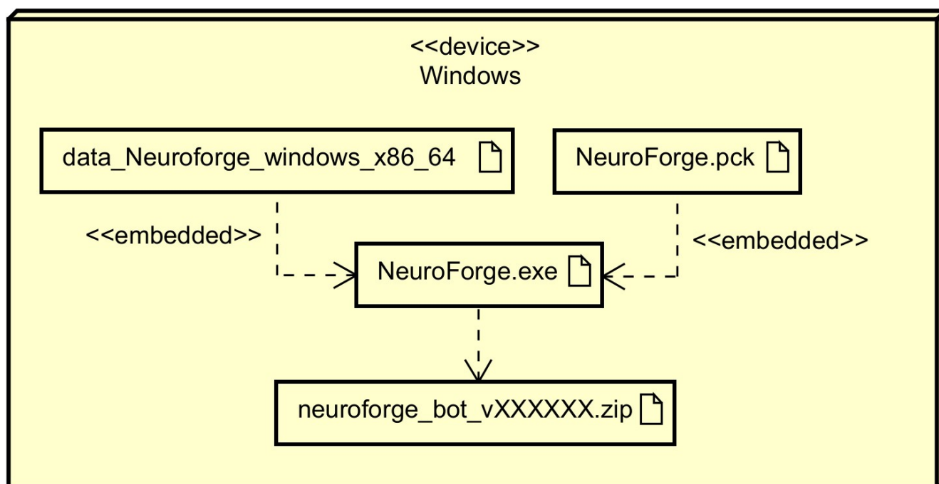
Figura 6.4: Diagrama de despliegue de NeuroForge.
