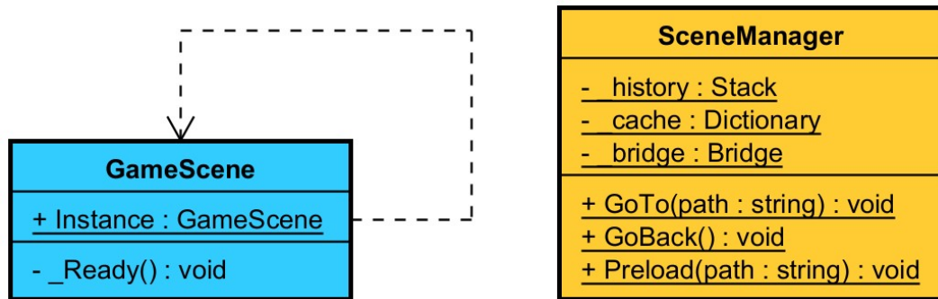
Figura 6.14: Patrón Singleton aplicado en GameScene y SceneManager .
