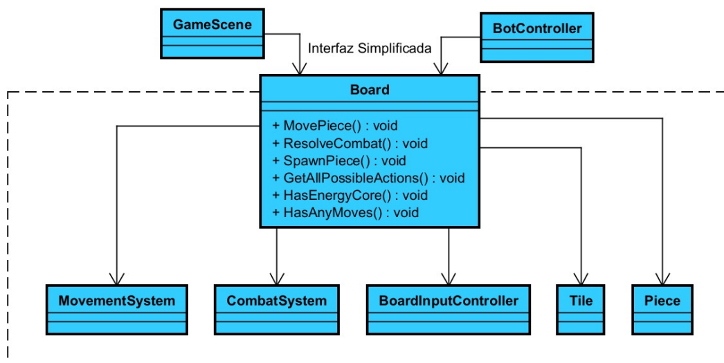
Figura 6.16: Patrón Fachada con Board como punto de acceso unificado al subsistema de tablero.
