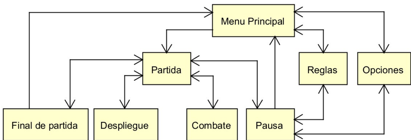
Figura 6.5: Diagrama de navegación de las interfaces de NeuroForge.
