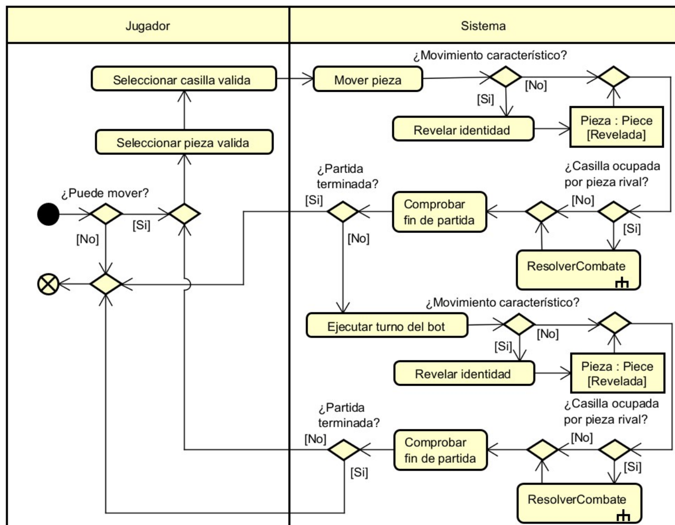
Figura 5.4: Diagrama de actividad: Jugar turnos
