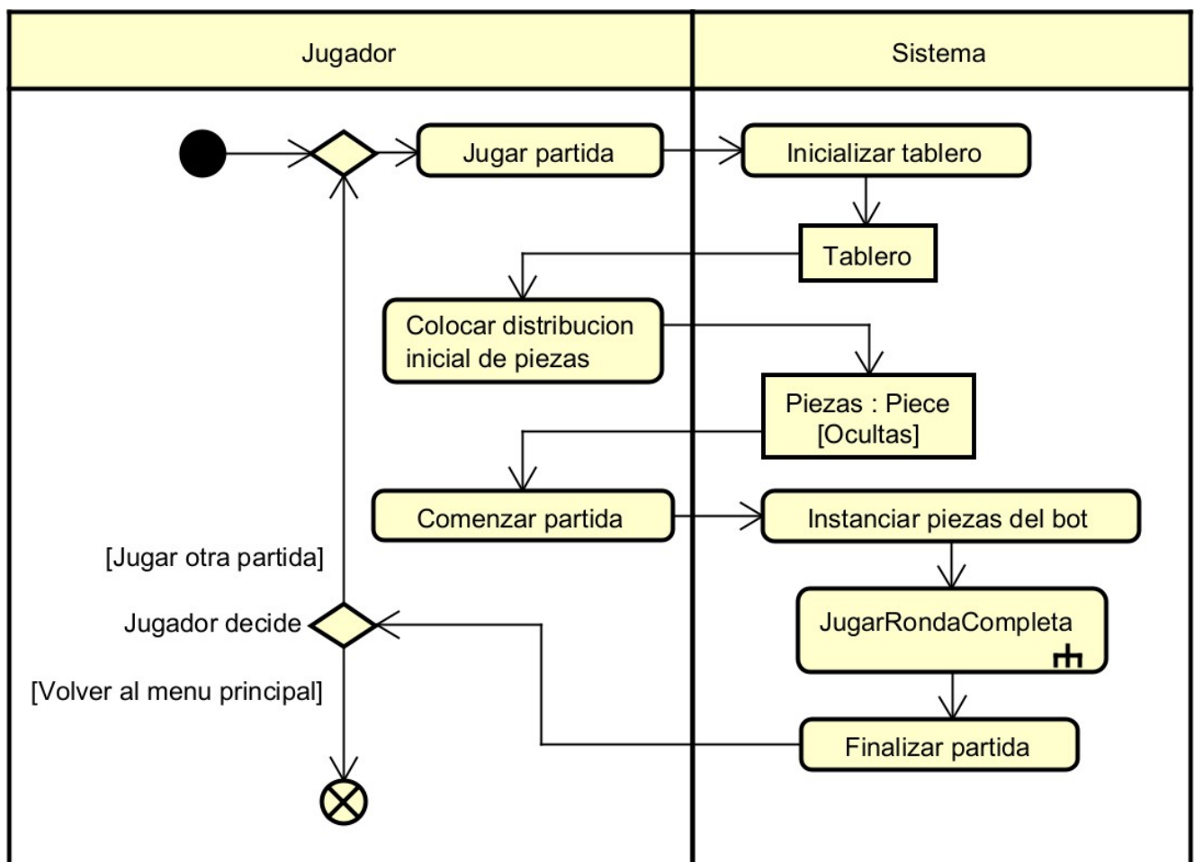
Figura 5.3: Diagrama de actividad: Jugar partida
