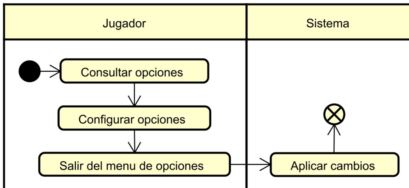
Figura 5.6: Diagrama de actividad: Consultar opciones
