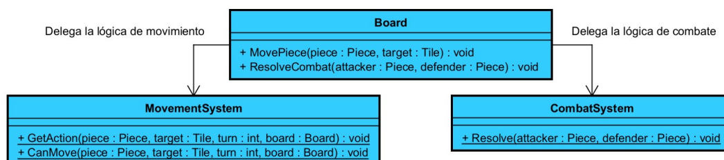
Figura 6.15: Patrón Strategy con MovementSystem y CombatSystem como estrategias delegadas desde Board .
