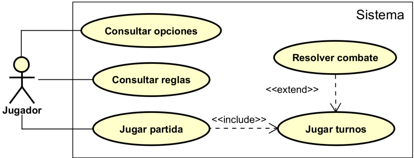
Figura 5.1: Diagrama de casos de uso
