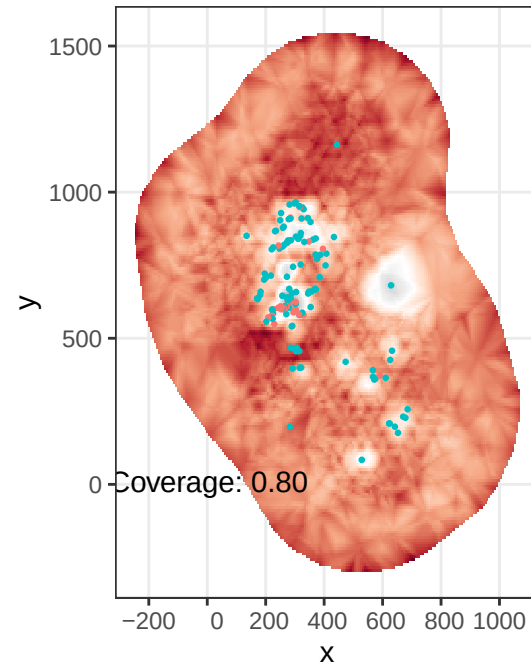
Posterior 97.5%
