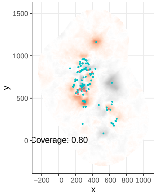
Posterior median
