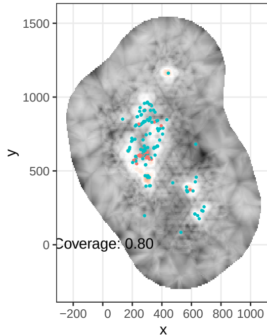
Posterior 2.5%
