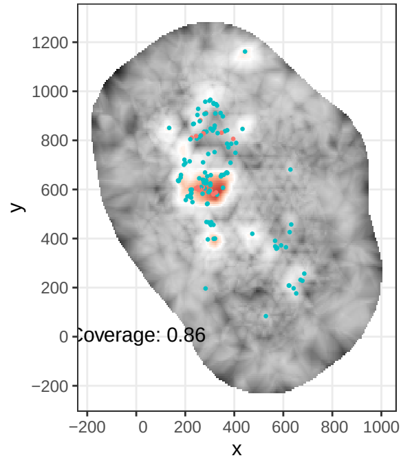
Posterior 2.5%
