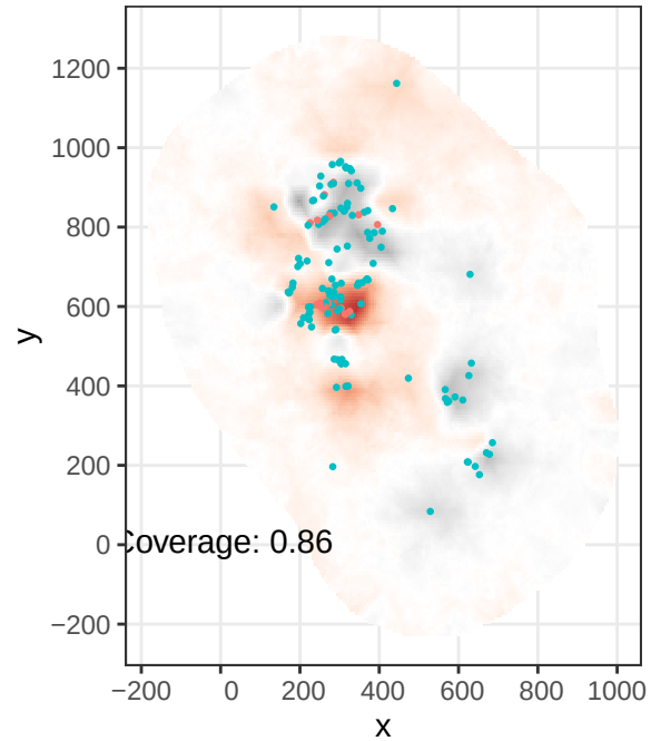
Posterior median
