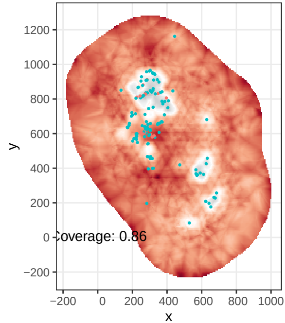
Posterior 97.5%
