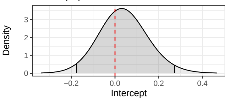
Intercept posterior
