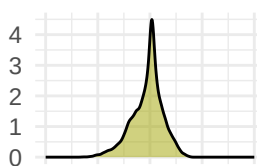
GB LM
