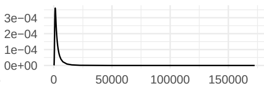
Precision for elev
