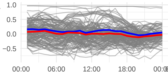
QM
