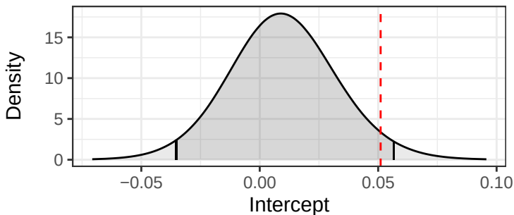
Intercept posterior
