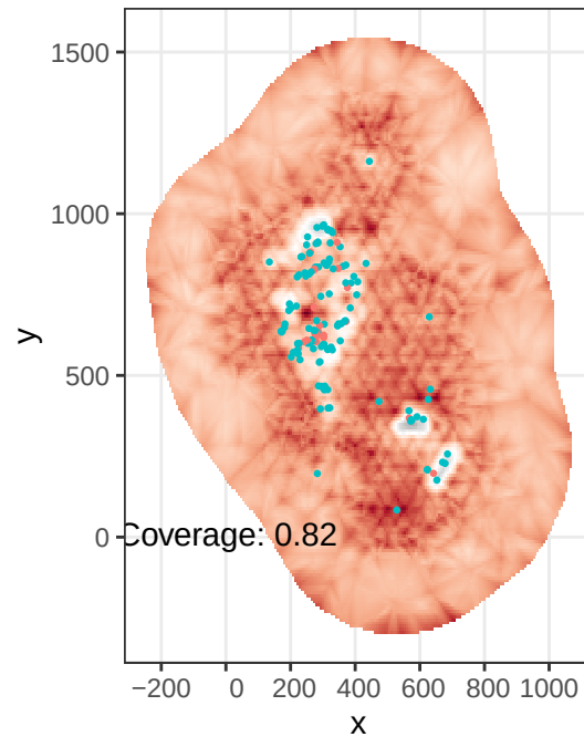
Posterior 97.5%
