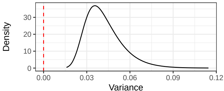
Intercept posterior
