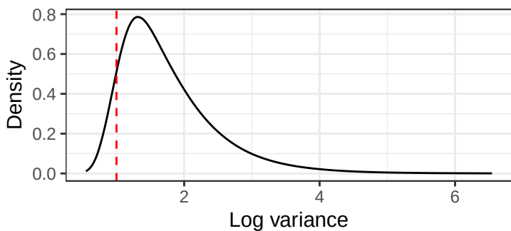
Variance posterior
